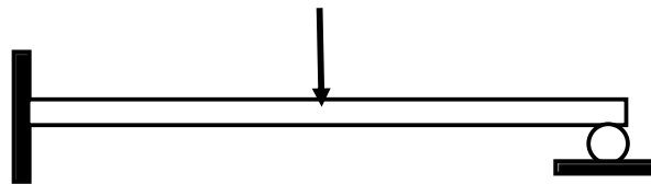
شكل ١ (خ) : كمرة كابولية مع دعامة منزلقة
