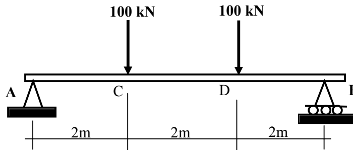
شكل ٩ (أ) - كمر بسيط - ٣٤ -
