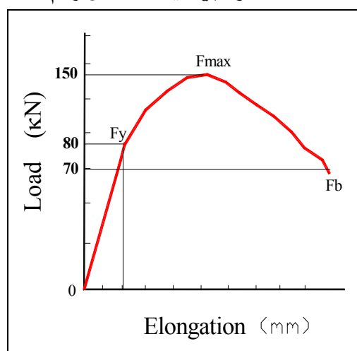
شكل ٥ : منحنى قوة الشد والاستطالة
