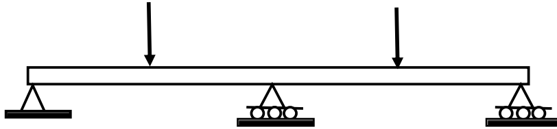
شكل ١ (ب) : كمر مستمرة Continuous Beam
