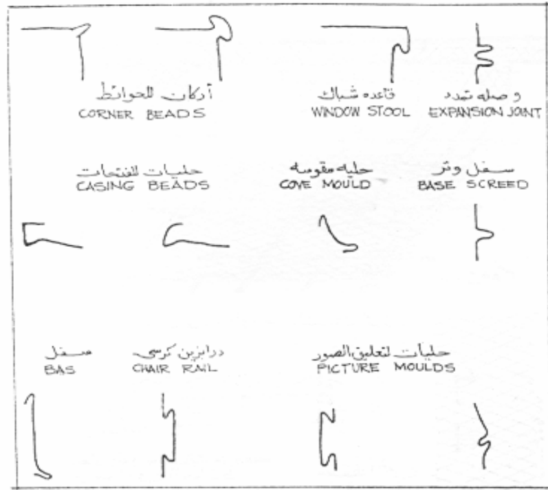
٢) الطروفيات المعدنية للبياض METAL TRIM SHAPES FOR PLASTER
