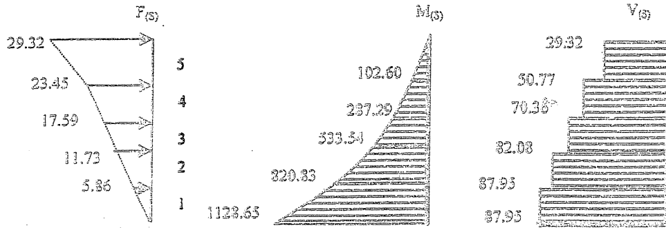
الشكل (٧) - مخططي عزم الانحناء ( M_s ) وقوى القص ( V_s ) المطبقة على الجدار القصي رقم (١)
