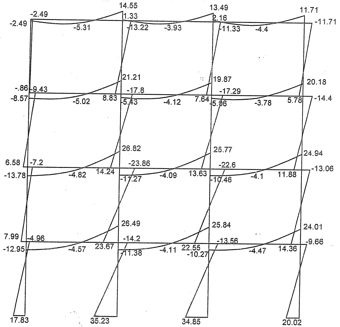
Frame F2 Bending Moment U3
