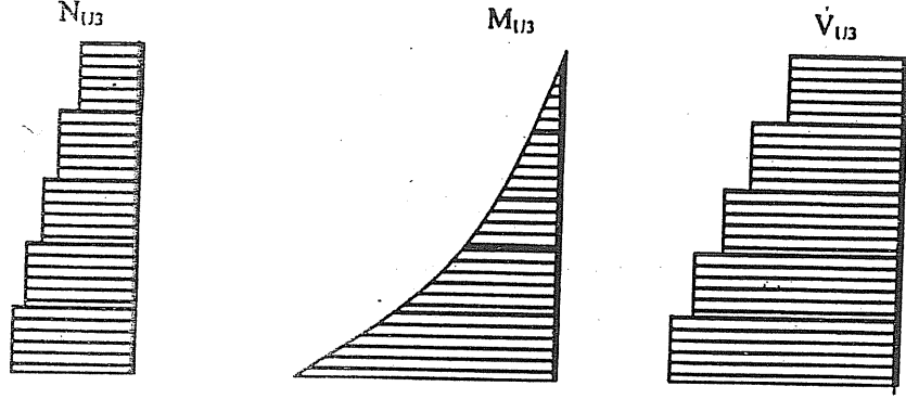
الشكل (١٠) - القوى الداخلية وعزوم الانعطاف الحدية لحالة التحميل ( U_3 )
