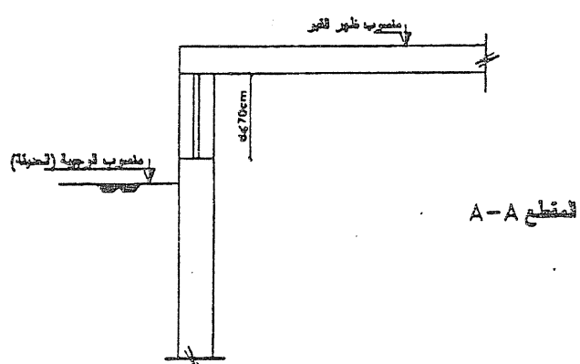
الشكل رقم (١) اشتراطات النوافذ في الجدران المحيطة في القبو
