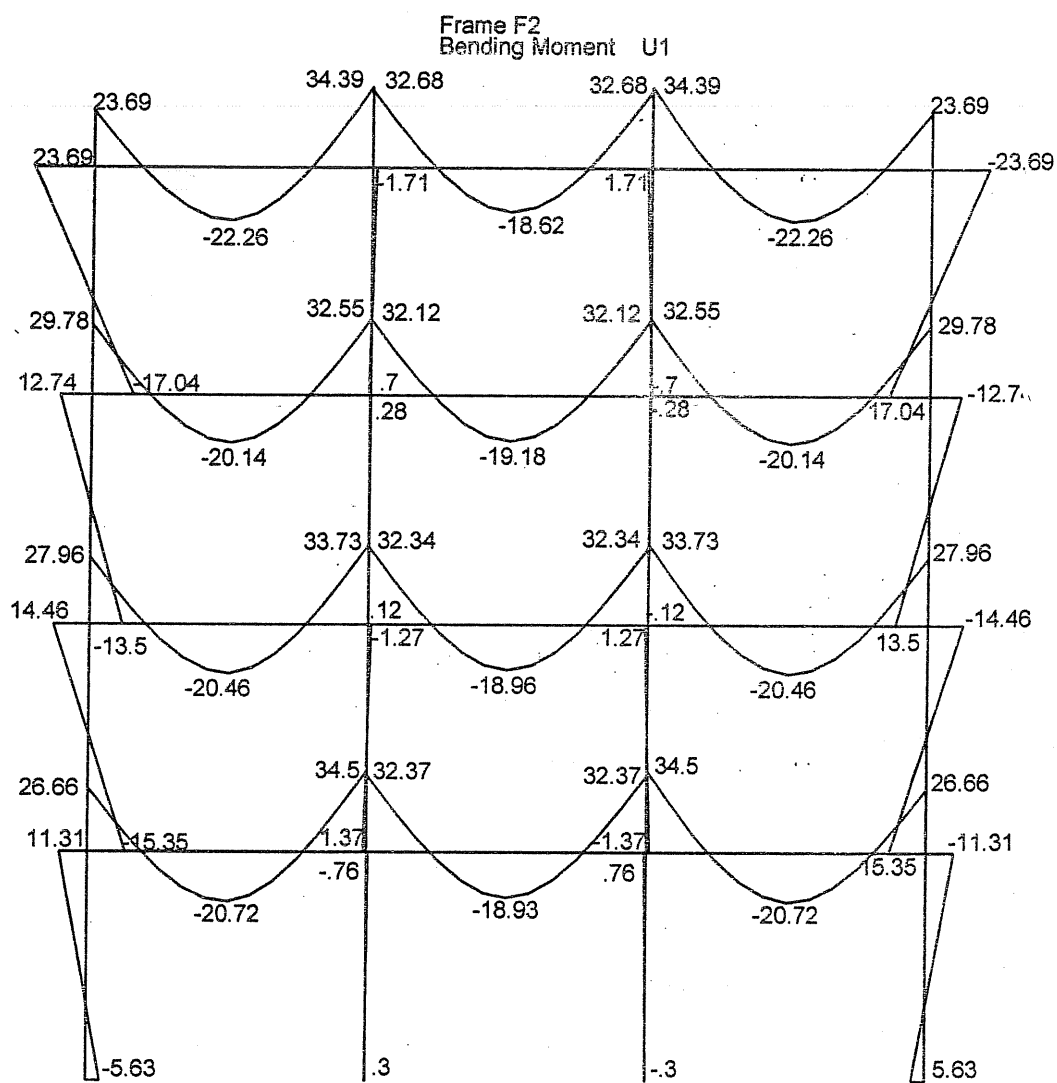
مخطط العزم للإطار الداخلي F2 حالة التركيب U1
