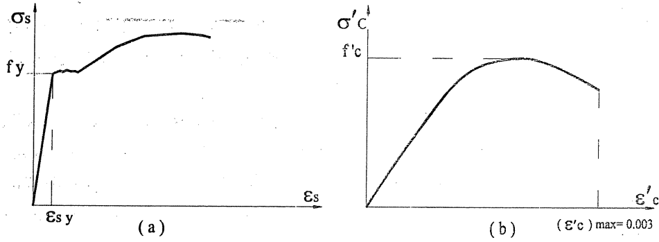
الشكل رقم (٣) مخططات الإجهاد - الانفعال للبيتون والفولاذ
