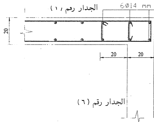
الشكل رقم (٨) تفاصيل التسليح في الجدار رقم ٢/٠
