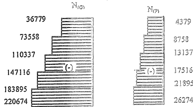
الشكل (٦) - مخططي القوى النافذية الميتة ( N_g ) والحية ( N_p ) للجدار القصي رقم (١)
