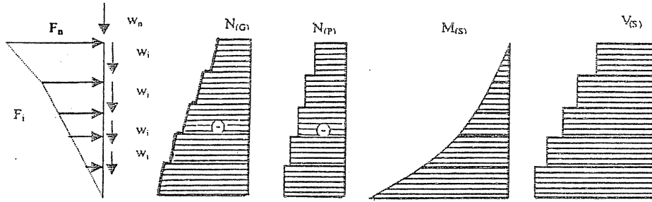
الشكل (٤): مخططات القوى الناعمة وعزوم الانعطاف وقوى القص المطبقة على الجدران القصية
