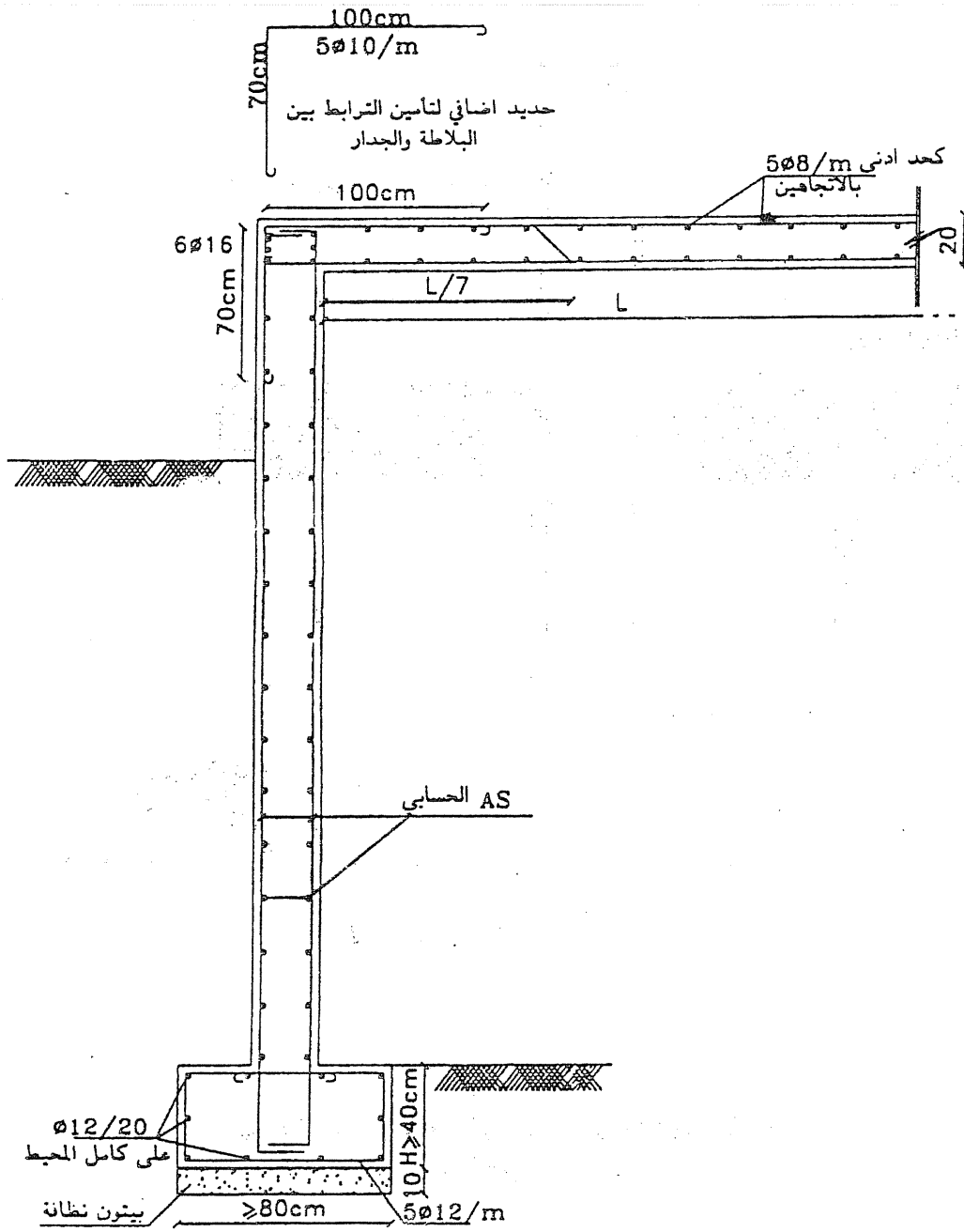
تفصيلة رقم (٤)
