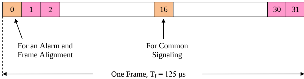
الشكل (٦ - ٩): إطار نظام الحامل الرقمي "E1"
