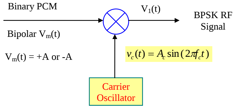
الشكل (٨ - ١٨): توليد إشارة "BPSK"
