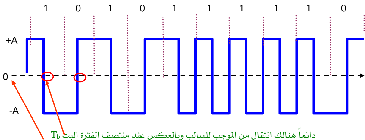
الشكل (٧- ١٤): ترميز مانشستر كود
