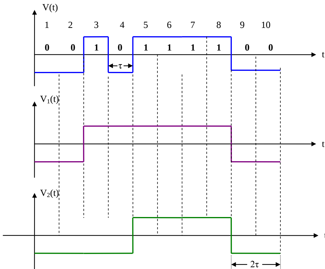
الشكل (٨ - ٢٧): حل مثال (٨ - ٧)
