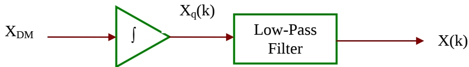
الشكل (٥-٨): فك تعديل دلتا
