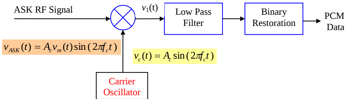
الشكل (٨- ١١): الكشف المترابط لإشارة "ASK"
