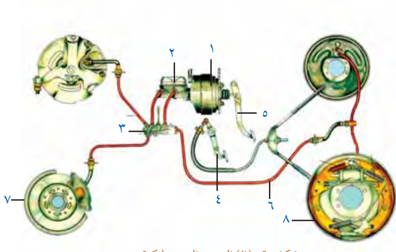
شكل رقم (٢) الوحدة الهيدروليكية
