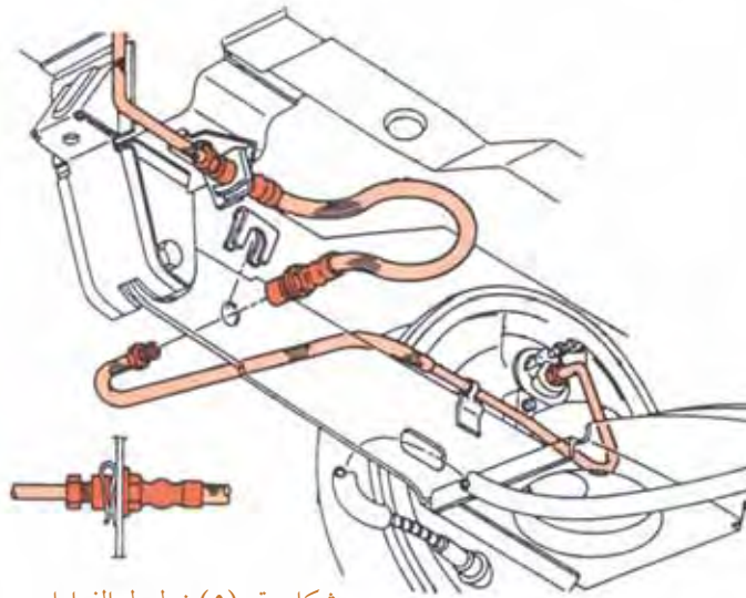
شكل رقم (٥) خطوط الفرامل
