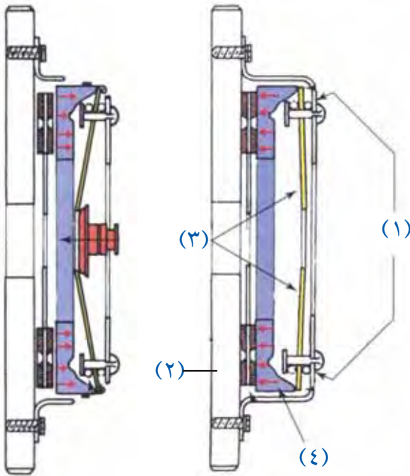
الشكل (١١-أ) وضع الفصل
