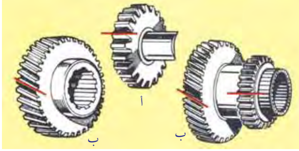
شكل رقم (١) تروس ذات أسنان مستقيمة وأسنان مائلة
