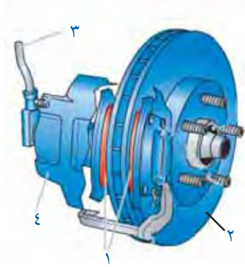
شكل رقم (٣) أجزاء فرامل القرص
