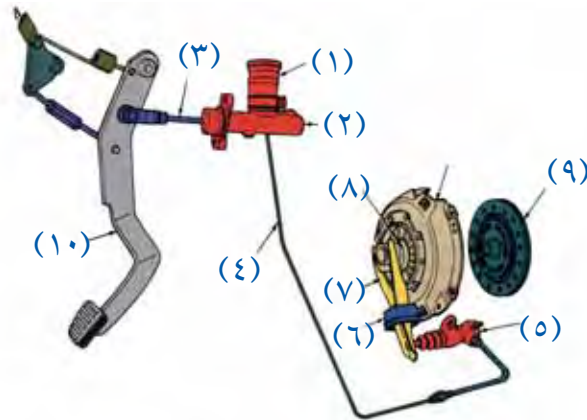
الشكل (٨) الوصلة الهيدروليكية
