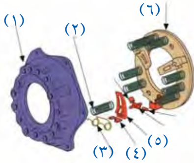
الشكل ( ١ ) القابض ذو النوابض اللولبية
