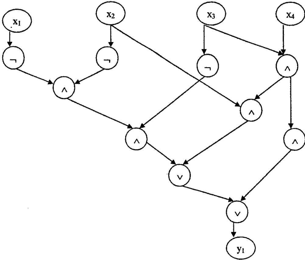
شكل (10-1) يبين دارة منطقية بسيطة تعتمد على القاعدة القانونية فيها D(\alpha)=6 و Z(\alpha)=15
