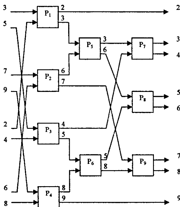
الشكل (11-3) شبكة دمج من أجل حجم المتسلسلتين n=4
