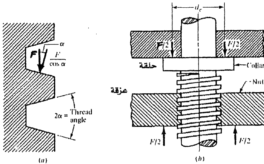
شكل (7-6) (a) أثر القوة العمودية على السن الأكم
