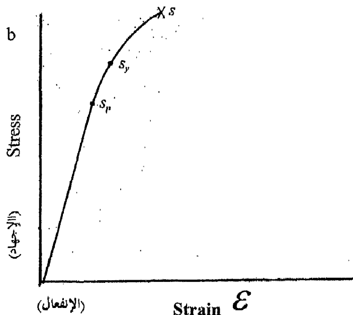
(15- 6) منحنى (الإجهاد - الإنفعال) لمعدن برغي
