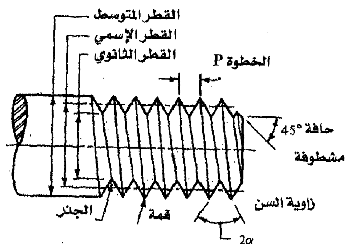
شكل (1-6) المصطلحات الفنية للبراشي
