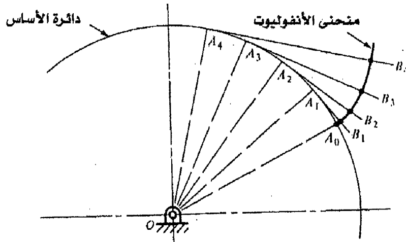
شكل (8-5) إنشاء منحنى الإنفولتيوت.
