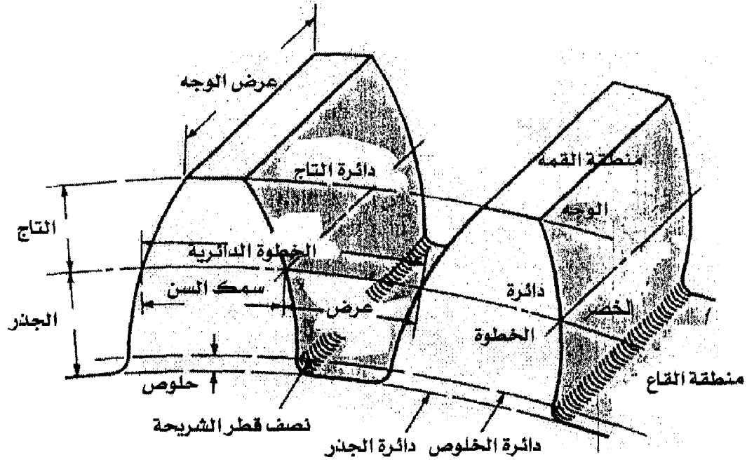
شكل (5-5) مصطلحات خاصة بالترس العديل.
