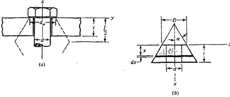
شكل (14- 6) توزيع قوى الضغط في عضو الوصلة
