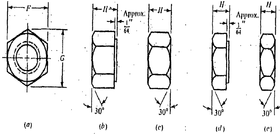
شكل (11-6) أنواع مختلفة من العزقات السداسية
