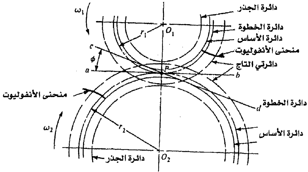
شكل (9- 5) رسم تخطيطي لزوج من التروس
