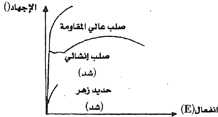
منحنى الإجهاد والانفعال لبعض المواد الهندسية
