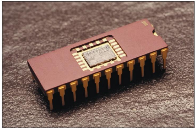
الشكل (5-10) الشريحة تتوضع على حوامل الشريحة
