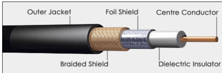
الشكل (4-8) الكابل المحوري
