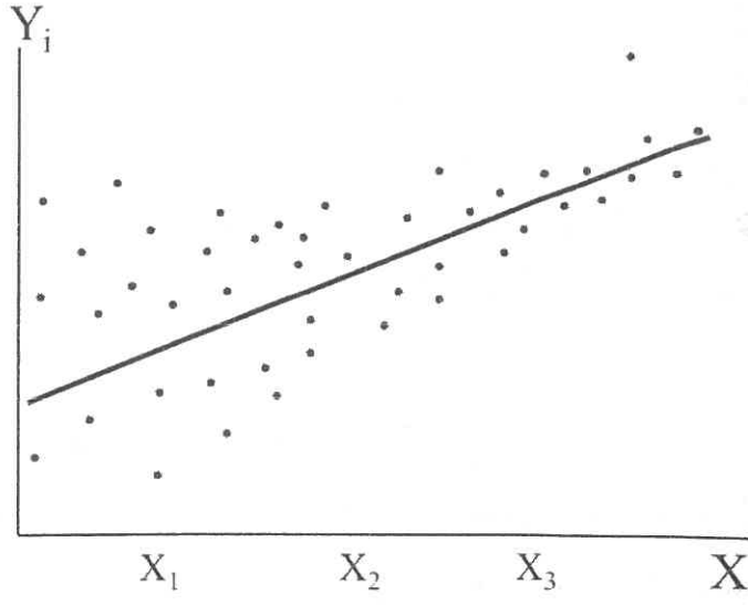
شكل رقم 6-3: مثال Heteroskedasticity بتباين متناقص
