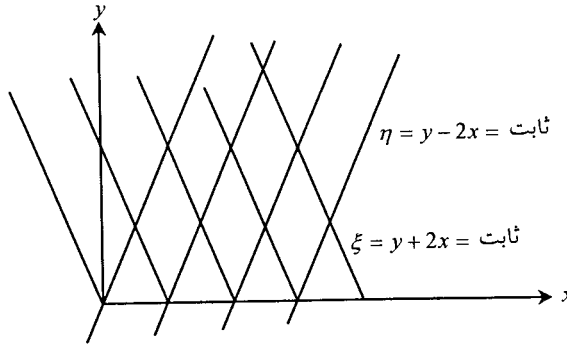
شكل 2-29 الإحداثيان الجديدان للمعادلة u_{xx} - 4u_{yy} + u_x = 0
