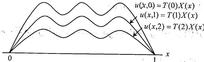
شكل 2-5 مخطط X(x)T(t) لقيمة مختلفة للزمن t
