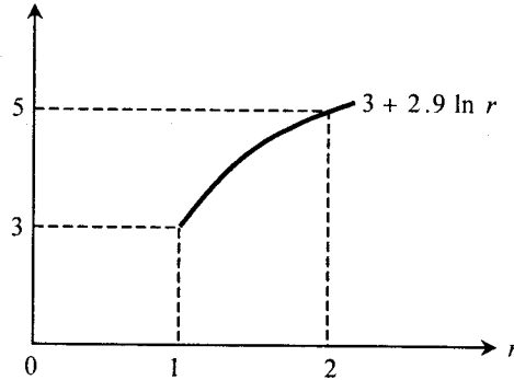
شكل 1-39 شريحة قطرية للجهد داخل الشكل الحلقي ( 1 < r < 2 )
