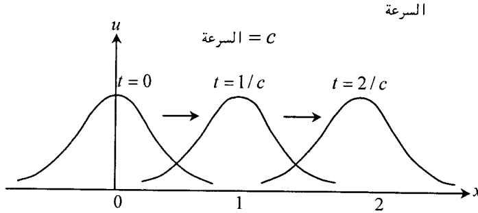
شكل 1-21 موجة متحركة إلى اليمين u(x, t) = e^{-(x-ct)^2}
