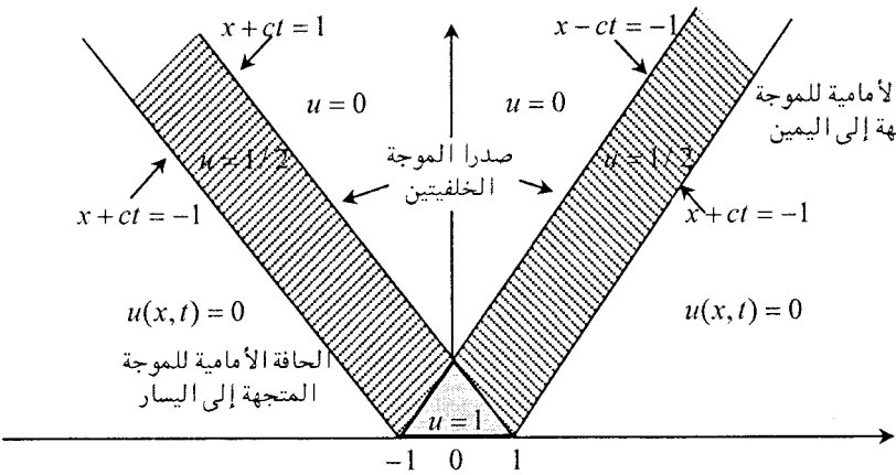
شكل 2-22 حل مسألة القيم الابتدائية (1) في المستوى xt
