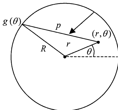
شكل 2-37 كمجموع مرجح جهود الحدود U(r, \theta)
