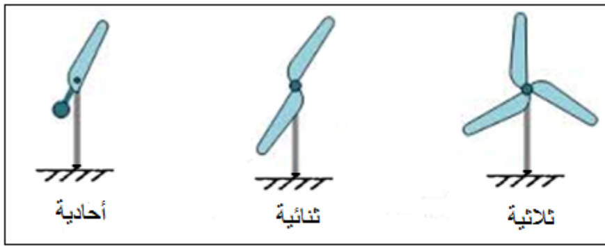
الشكل رقم (٢٧) : نماذج لتوربينات حسب عدد الريش
