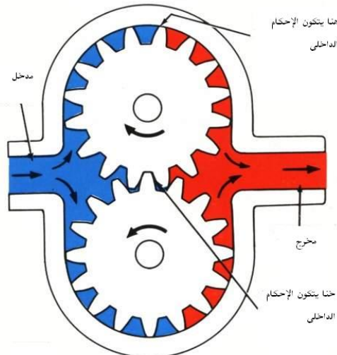
شكل ٦-٢ : مضخة ترسية خارجية فى التشغيل
