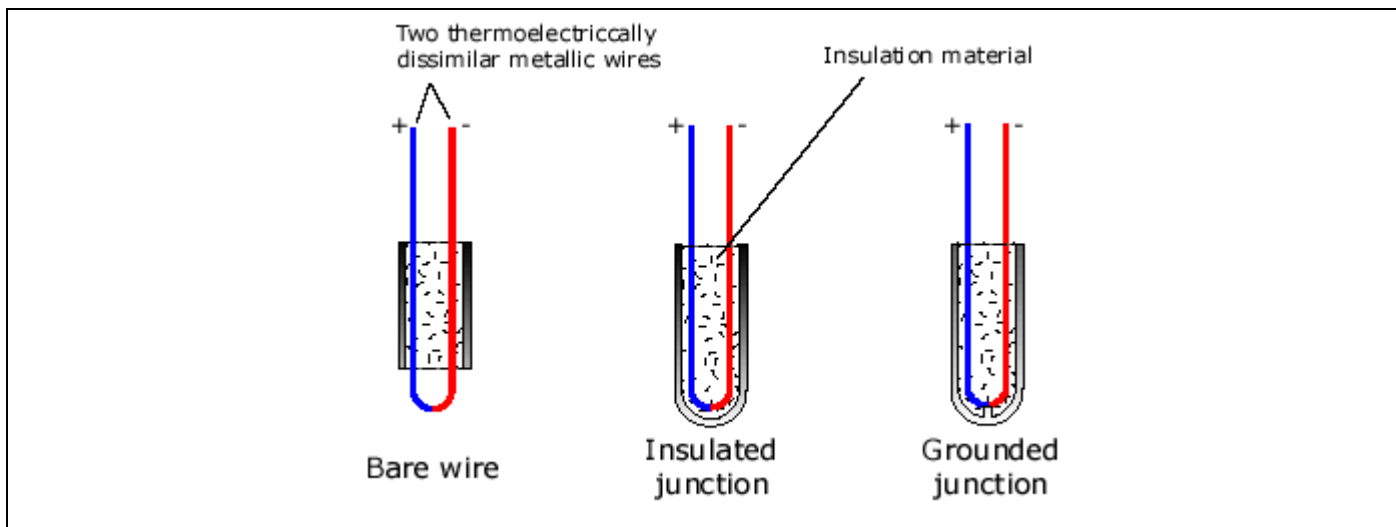
شكل (٣- ١) مزدوجات حرارية شائعة الاستخدام Typical Thermocouples
