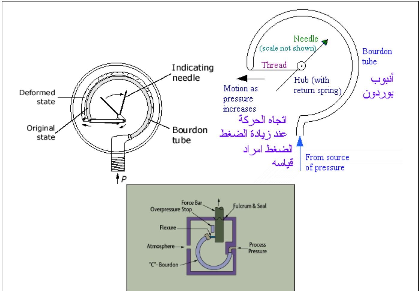
شكل (٢- ٣) تصاميم مختلفة لأنبوبة بوردون المستخدمة لقياس الضغط
