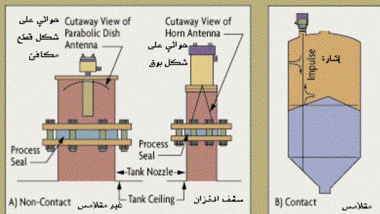
Radar-Based Antenna Installations طرق مختلفة لاستخدام أشعة الرادار لقياس مستوى السوائل
