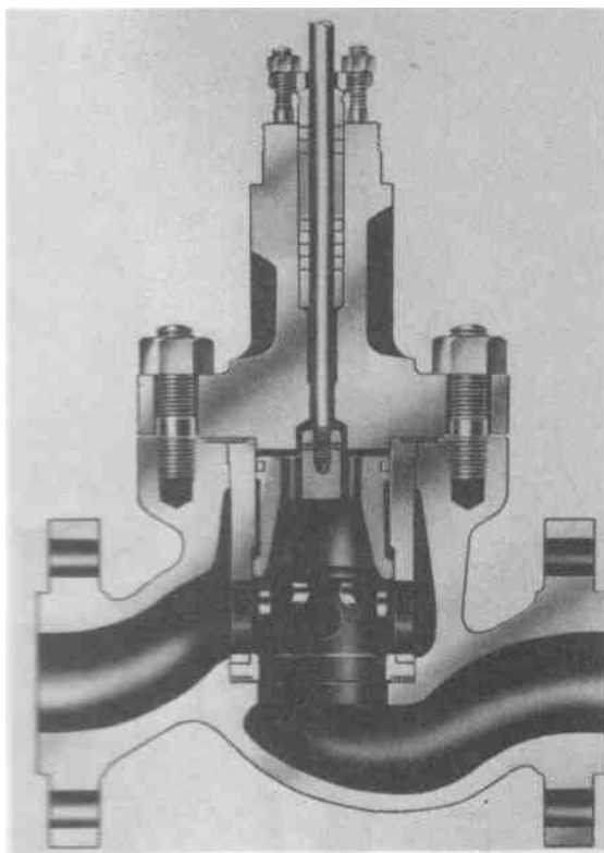
شكل (٧-٤) صمام قفص
