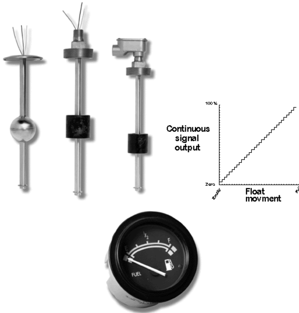
شكل (٤ - ٨) نظام لتحديد مستوى سائل بصورة مستمرة لترسل الإشارة إلي أجهزة التحكم Liquid level sensors with a continuous output signal for process control signal data
