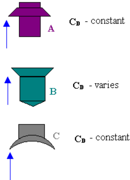
شكل (٤ - ٣) أشكال العوامات الشائعة الاستخدام ومعامل خروج المائع
