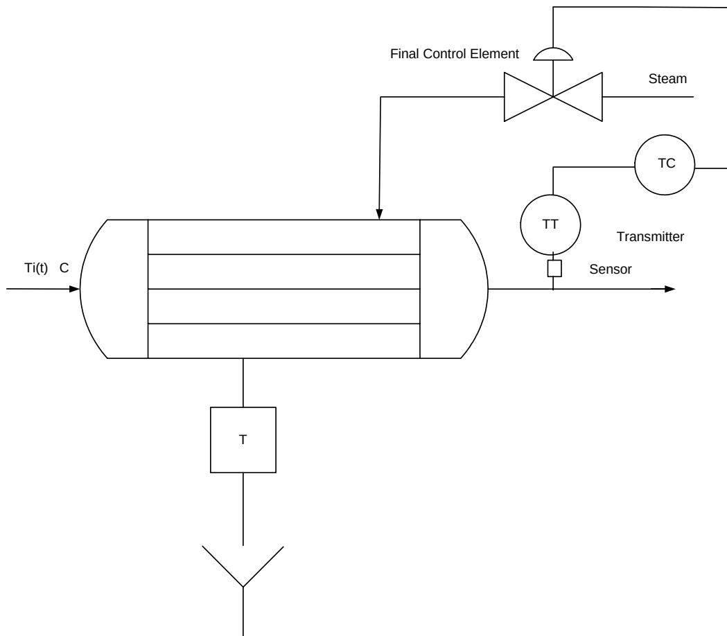
شكل (٥ - ٧) نظام التحكم في مبادل حراري
