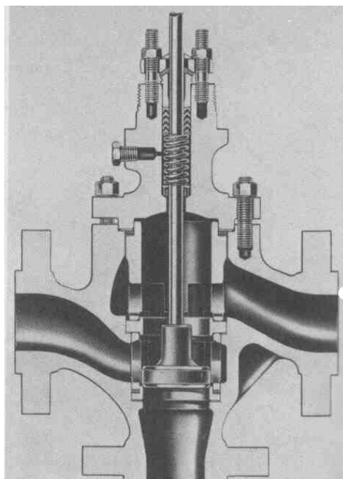
شكل (٧-٥) صمام ثلاثي الاتجاهات
