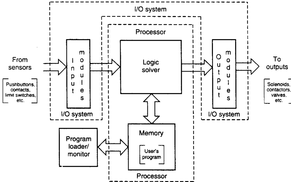
شكل (٦ - ٨) مخطط صندوقي لأجزاء المنظمات المنطقية المبرمجة
