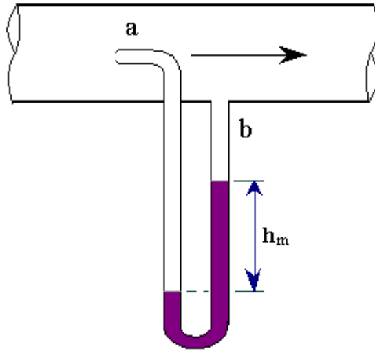
شكل (٤ - ٤) أنبوب بيتوت
