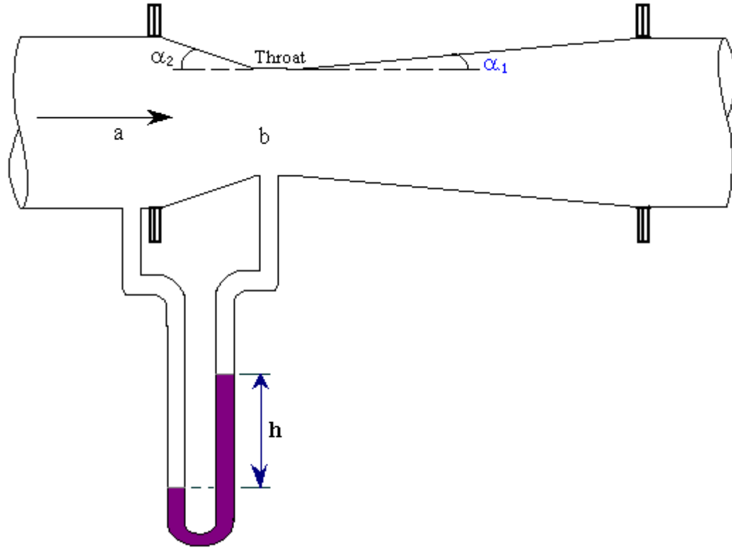
شكل (٤ - ١) أنبوبة فنشوري
