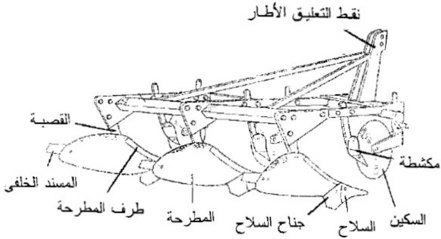
شكل (٨-٣). أجزاء المحراث القلاب
