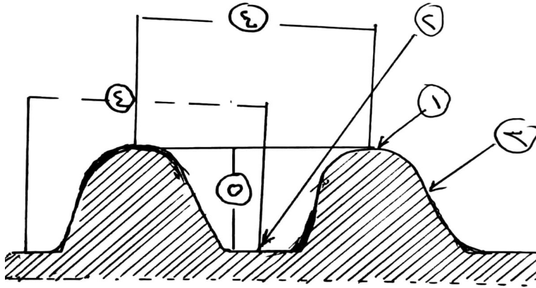
شكل (٨-١٧). أجزاء الخط (١) ظهر الخط، (٢) بطن الخط، (٣) الريشة، (٤) عرض الخط، (٥) ارتفاع الخط
