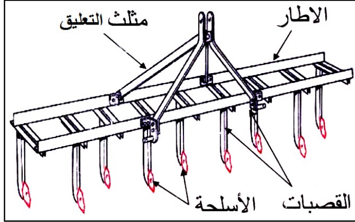
شكل (٨-٢). محراث حفار معلق ذو قصبات مرنة
