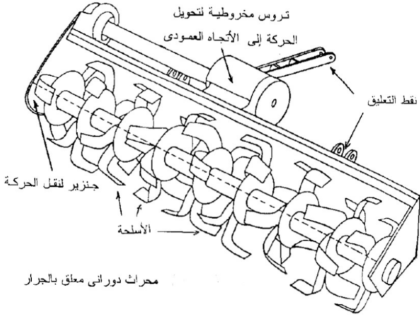
شكل (٦-٨). المحراث الدوراني
