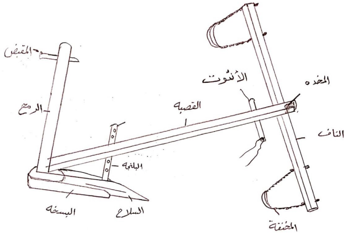
شكل (٨-١). أجزاء المحراث البلدى
