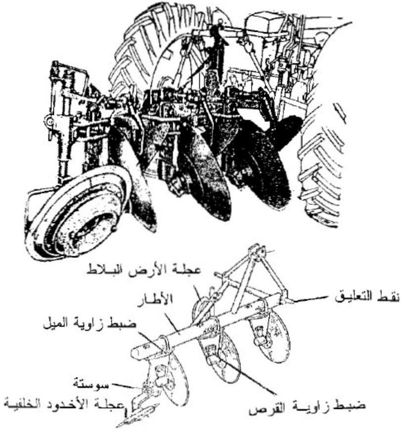
شكل (٨-٤). المحراث القلاب القرصي
