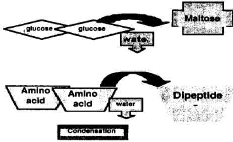
شكل (٣) تفاعل التكثيف
