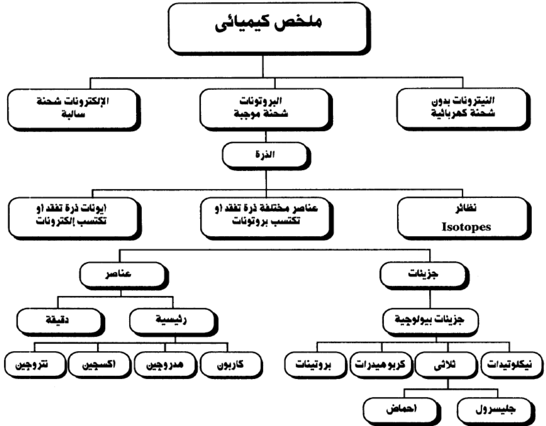
شكل (1) ملخص كيميائي
