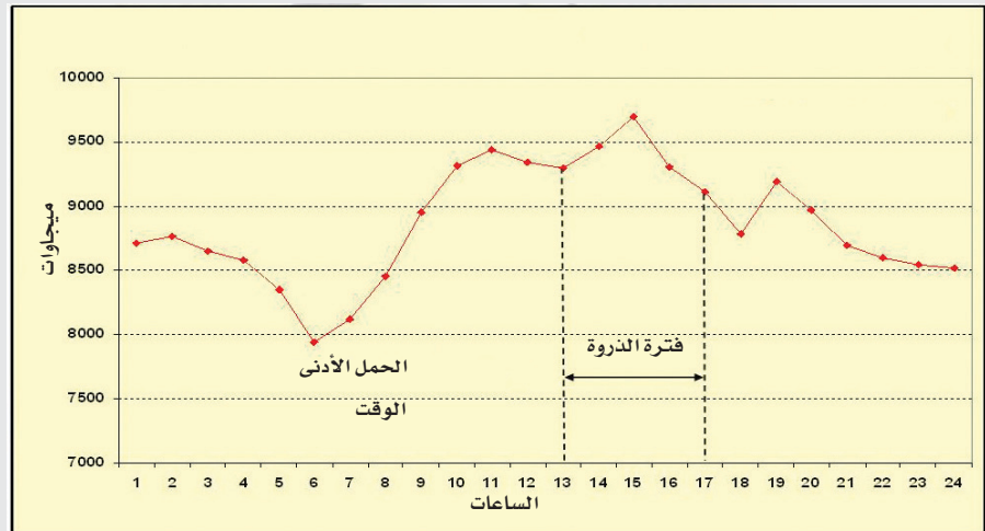
■ رسم بياني يوضح منحنى الأحمال اليومية لمشاركة المنطقة الوسطى بالملكة لعام ٢٠٠٦م.
