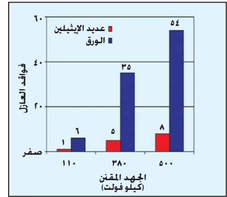
■ شكل (١) العلاقة بين فوائد العزل والجهد المثقن.
