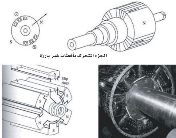
الجزء المتحرك بأقطاب بارزة
