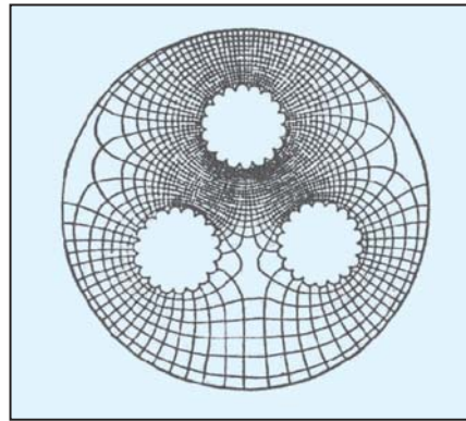
■ المجال الكهربائي لكابل ثلاثي القلوب محاط بحاجب معدني.
