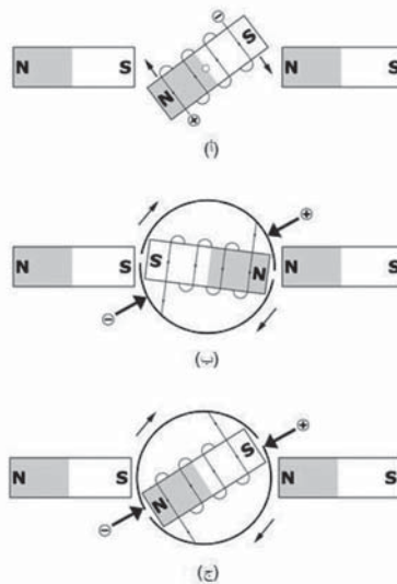
■ شكل (٧) كيفية عمل محرك تيار ثابت.
