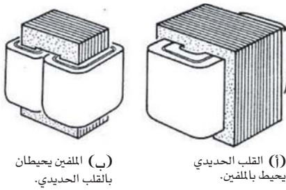
شكل (٥) طرق مختلفة لتصنيع المحولات.
