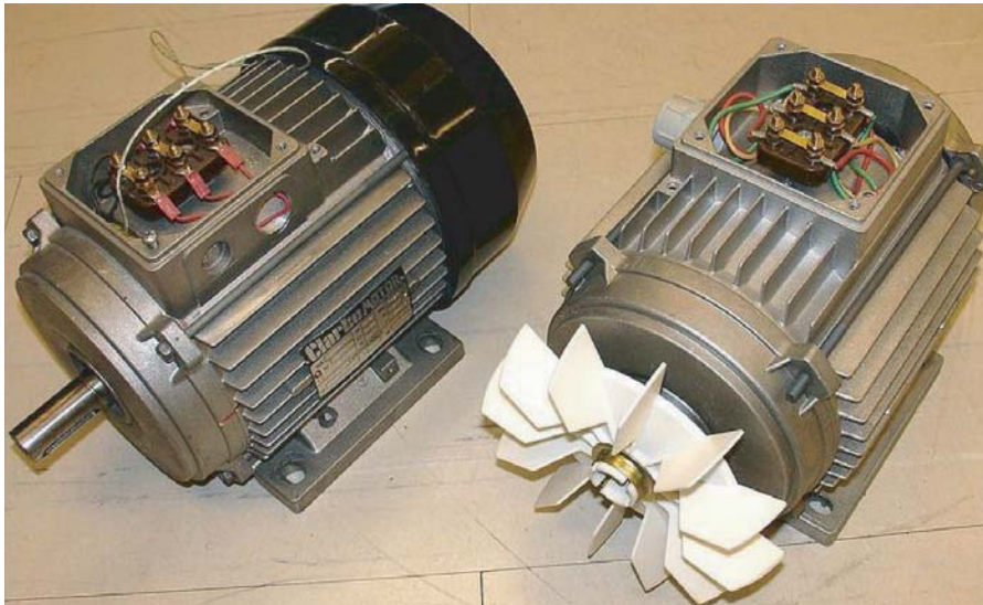
■ نموذجان للمحركات الحثية.
