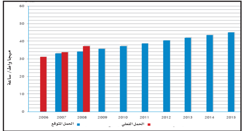
■ شكل (١٣) الأحمال الذروة الفعلية والمتوقعة في المملكة (٢٠٠٦م - ٢٠١٥م).
