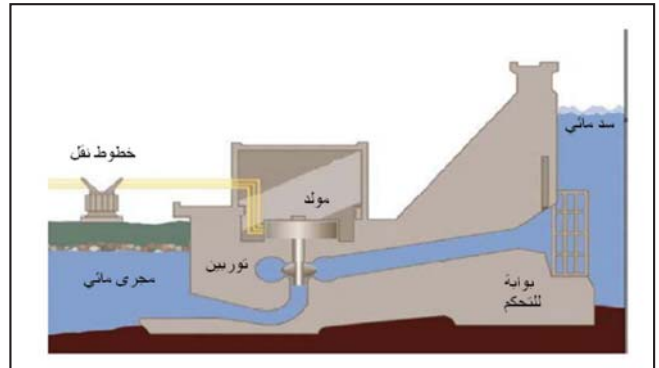
■ شكل (٨) استخدام السد المائي في إنتاج الكهرباء.
