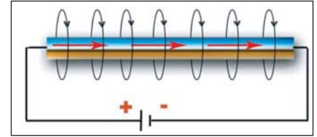
شكل (٢) المجال المغناطيسي الناتج عن سلك يحمل تياراً كهربائياً.
