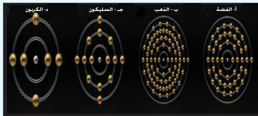
■ شكل (٣) مقارنة توصيلية بعض المواد من خلال ارتباط الإلكترونات بالنواة.
