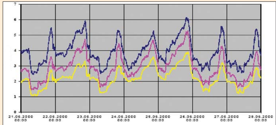
■ شكل (٨) مثال على التوافقيات الخامسة في نظم توزيع الكهرباء في النمسا على مستوى جهد مختلف من ٤٠٠ فولت و ٣٠ كيلوفولت و ١١٠ كيلوفولت على مدى أسبوع.
