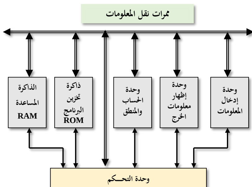
الشكل (22-1) : البنية الأساسية لأبسط نظام حاسبي
