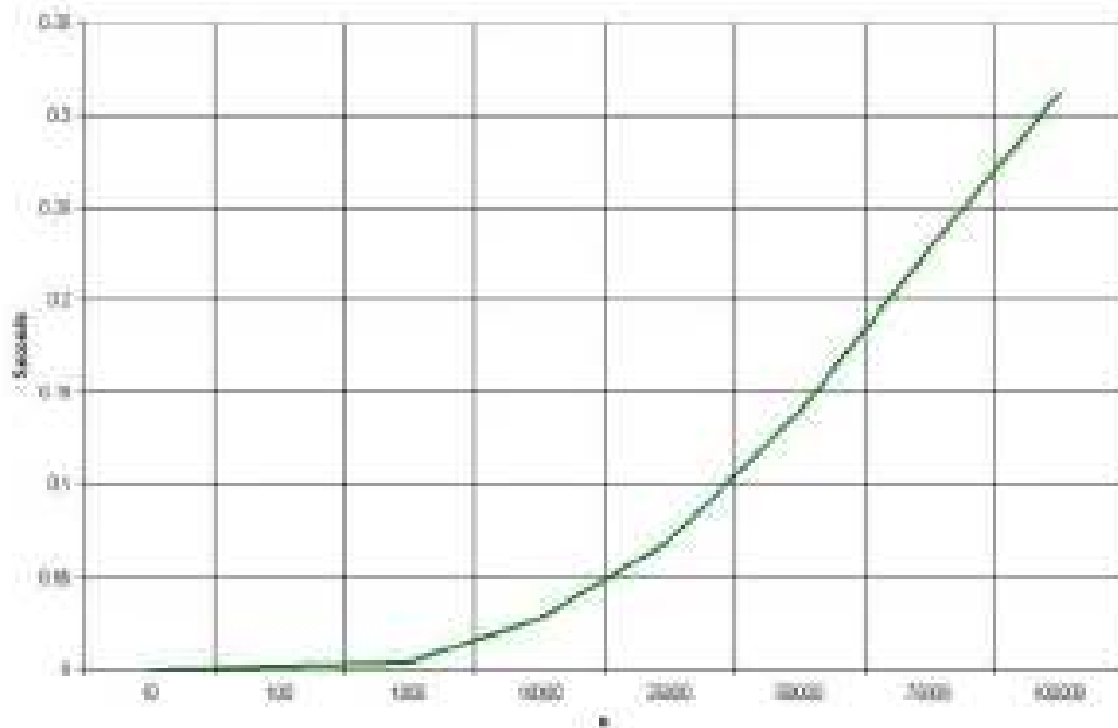
شكل(11):فعالية خوارزمية السريع (Quick Sort Efficiency)
