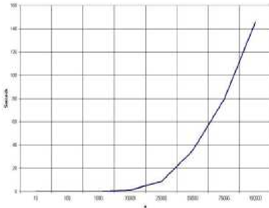
شكل (10): فعالية خوارزمية شيل (Shell Sort Efficiency)
