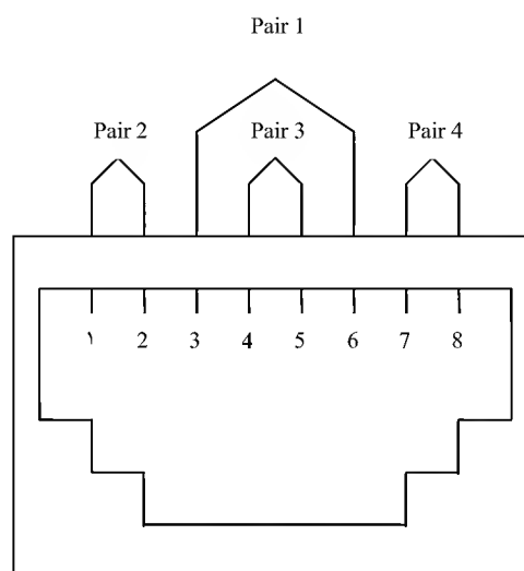
T568B
