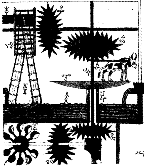
(شكل ١٠-١١) تصميم الجزارى لآلة رفع الماء. تصوير مخطوطة من "الكتاب في معرفة الحيل الهندسية"، لبدیع الزمان الجزارى - القرن الرابع عشر
