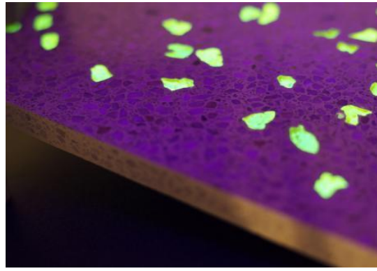
شكل (2.9): الاسمنت المضيء أو المشع (Luminous concrete)
