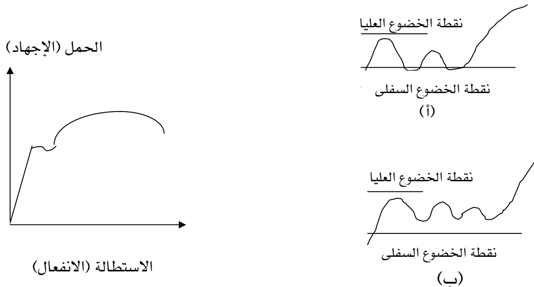
الشكل رقم ٦ : منحني الإجهاد والانفعال. (أ) و(ب) بيان منطقة الخضوع حسب النتائج.
