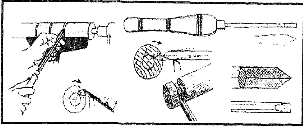
الشكل يبين المنقار واستخداماته
