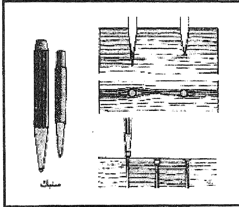
استخدام السمبك في ادخال المسمار تحت مستوى الخشب
