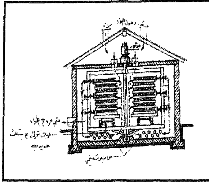
فرن التجفيف بالطريقة المزدوجة/ طريقة ماكنيل
