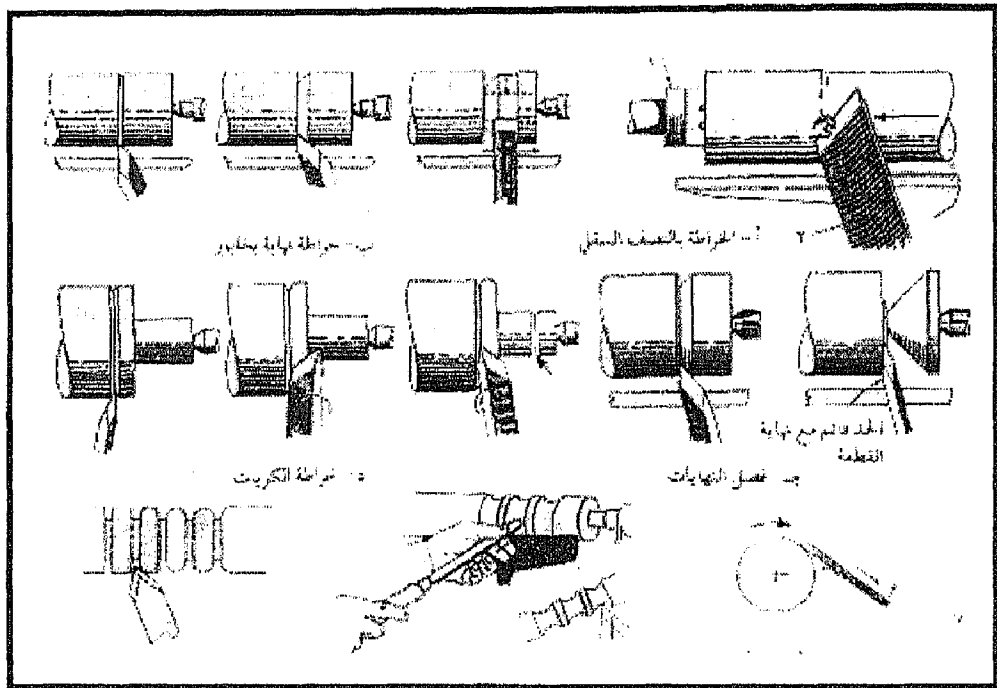
طريقة استخدام الاسلحة الحادة في عملية الخراطة
