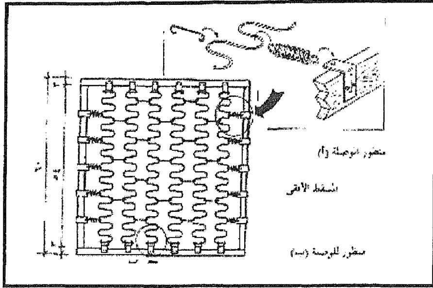
الزنبركات المتعرجة Zigzag
