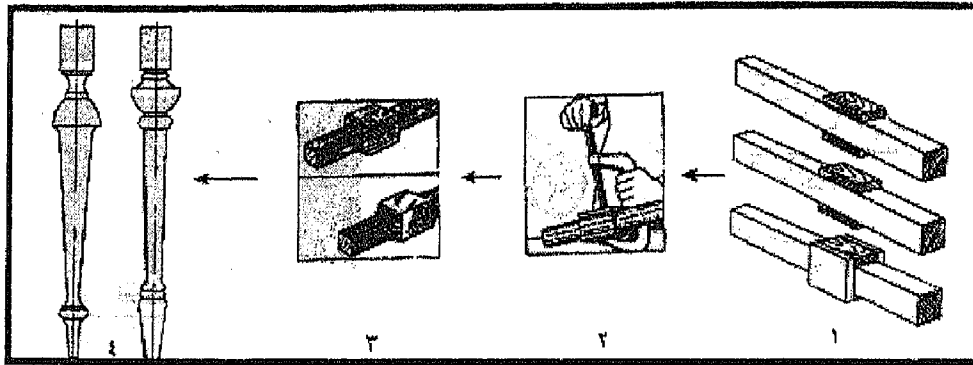
تجميع القطع الخشبية لخراطتها بالخرطة الاسطوانية
