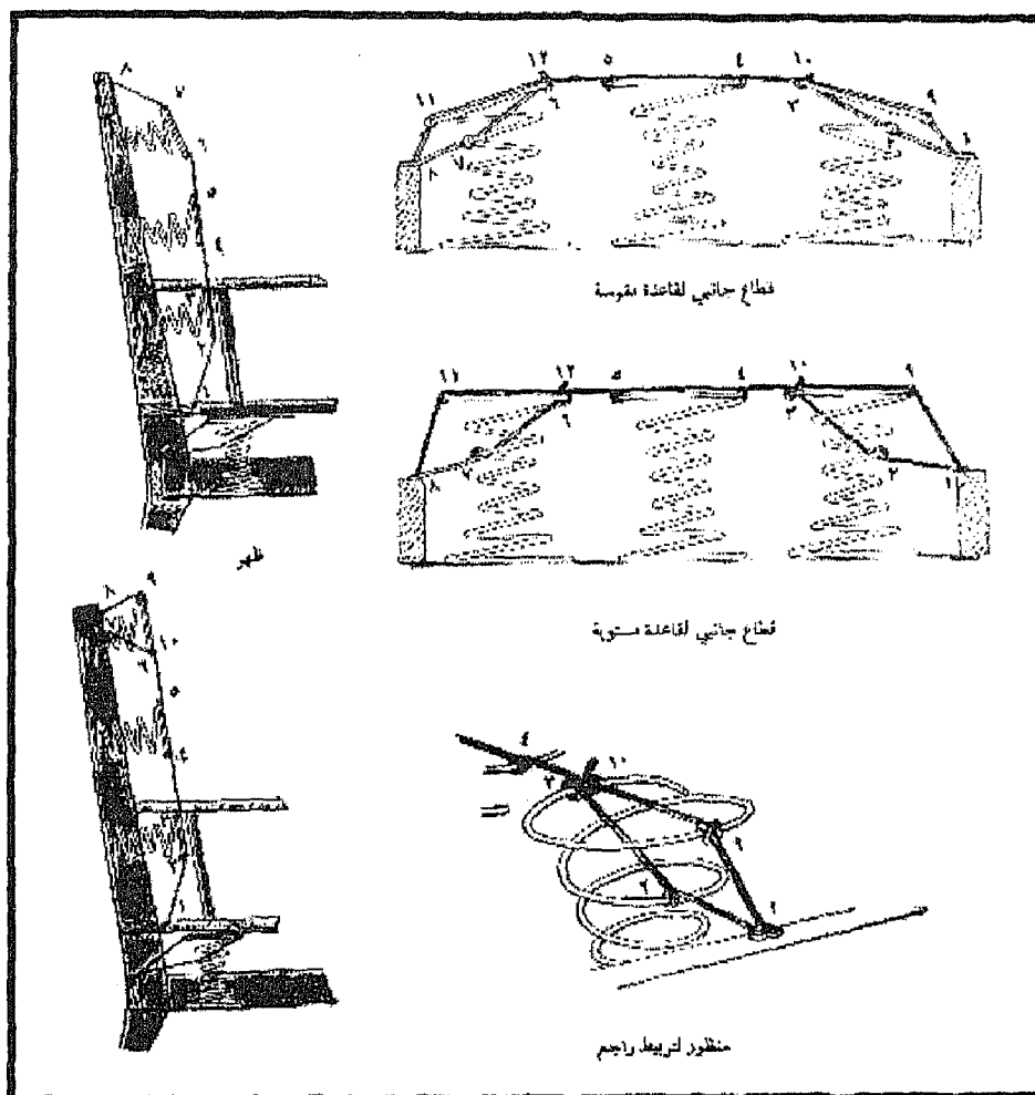
الزنبركات اللولبية في المقاعد والظهر
