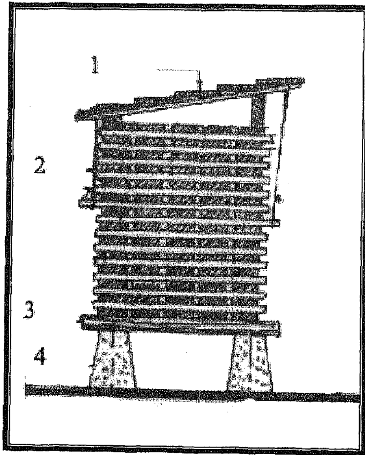
طريقة رص الواح الاخشاب تحت الجمالونات في التجفيف الطبيعي
