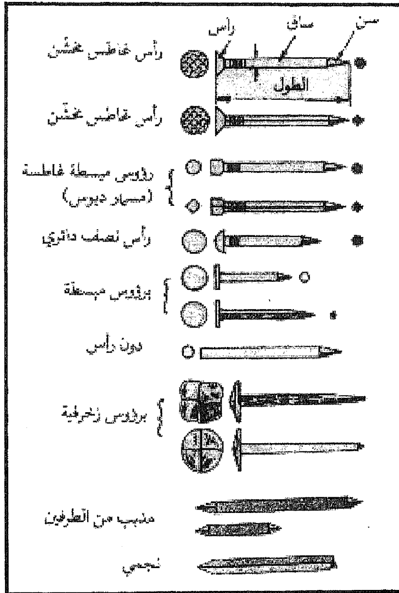
أنواع مختلفة من المسامير
