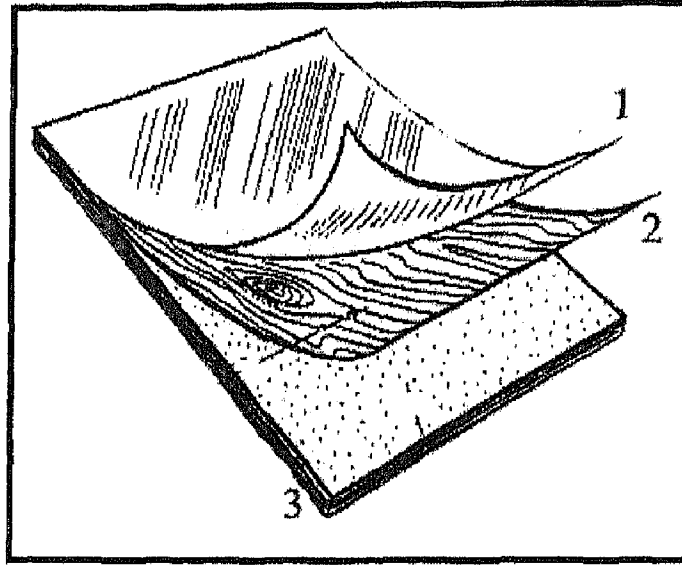
الشكل يوضح طبقات الفورمايكا
