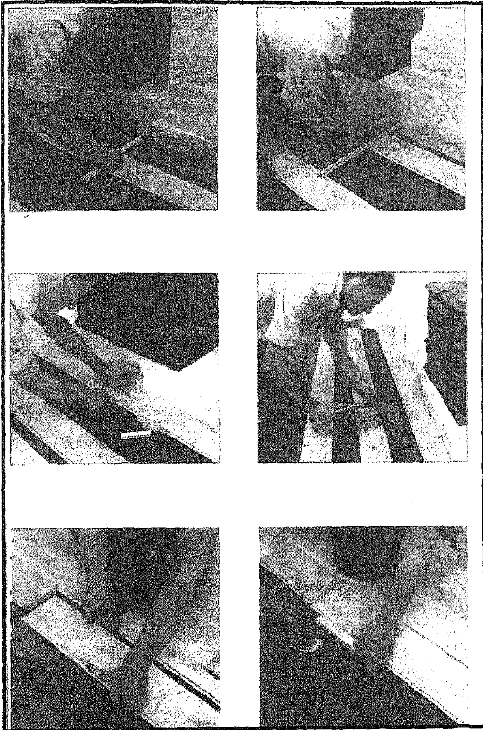
طريقة تجميع الشرائح الخشبية بالمجرى واللسان
