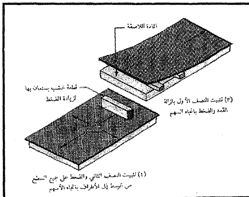
طريقة تركيب الفورمايكا باستخدام القدد أو البيش
