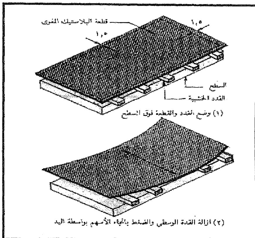
طريقة تركيب الفورمايكا باستخدام القدد أو البيش
