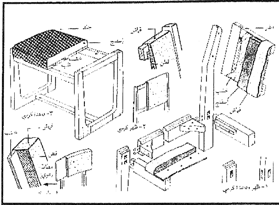
أجزاء وقطع التنجيد
