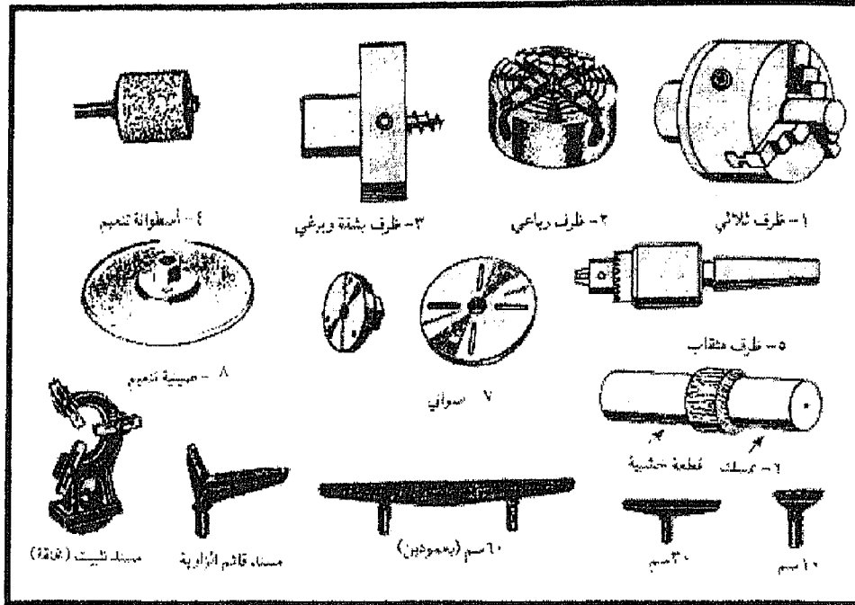
بعض اجزاء المخرطة وملحقاتها
