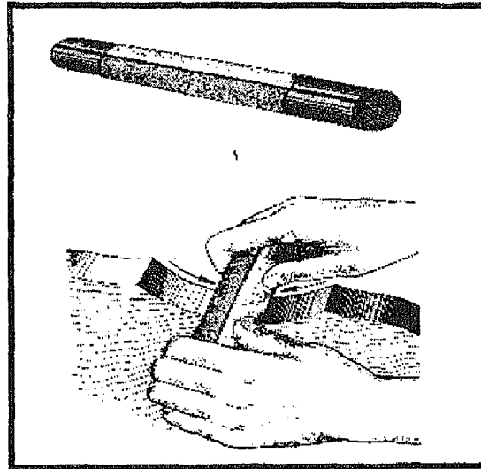
الطريقة الصحيحة لحف المنحنيات
