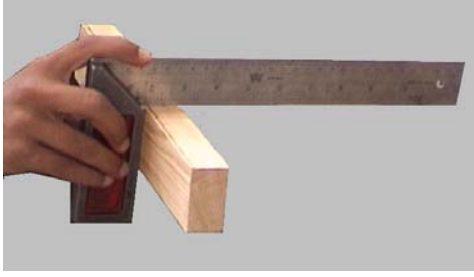
ب - التأكد من تعامد ودقة واستقامة الزاوية القائمة.
