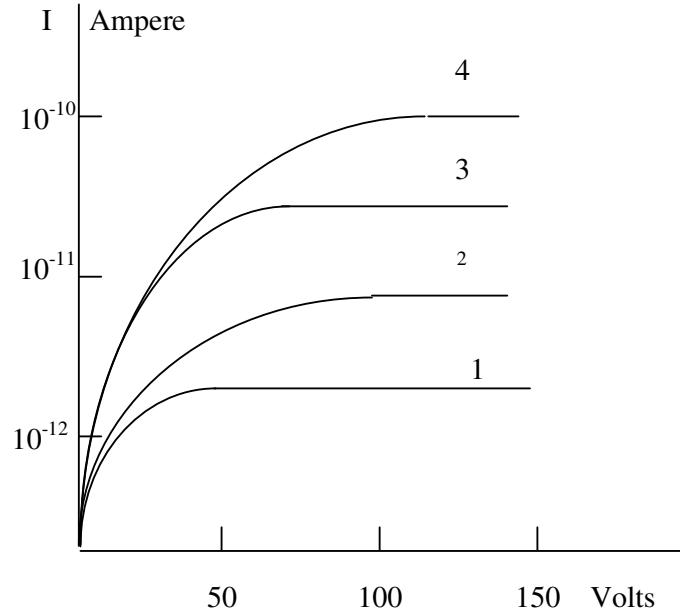
شكل (2-4): المميز الفولت أمبيرية لغرفة التأين
