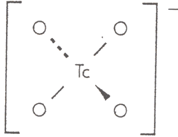
شكل (٩-٩): تركيب أيون برتكنيتيت التكنيشيوم ( \text{TcO}_4^- )
