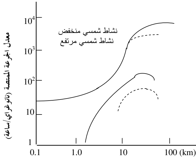
شكل (1-10) كيفية تغير مركبات الأشعة الكونية كدالة من الارتفاع عند خط عرض 50 درجة
