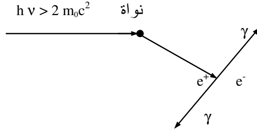
شكل (10-3) رسم توضيحي لعملية إنتاج الزوج الإلكتروني البوزيتروني ثم فناء البوزيترون
