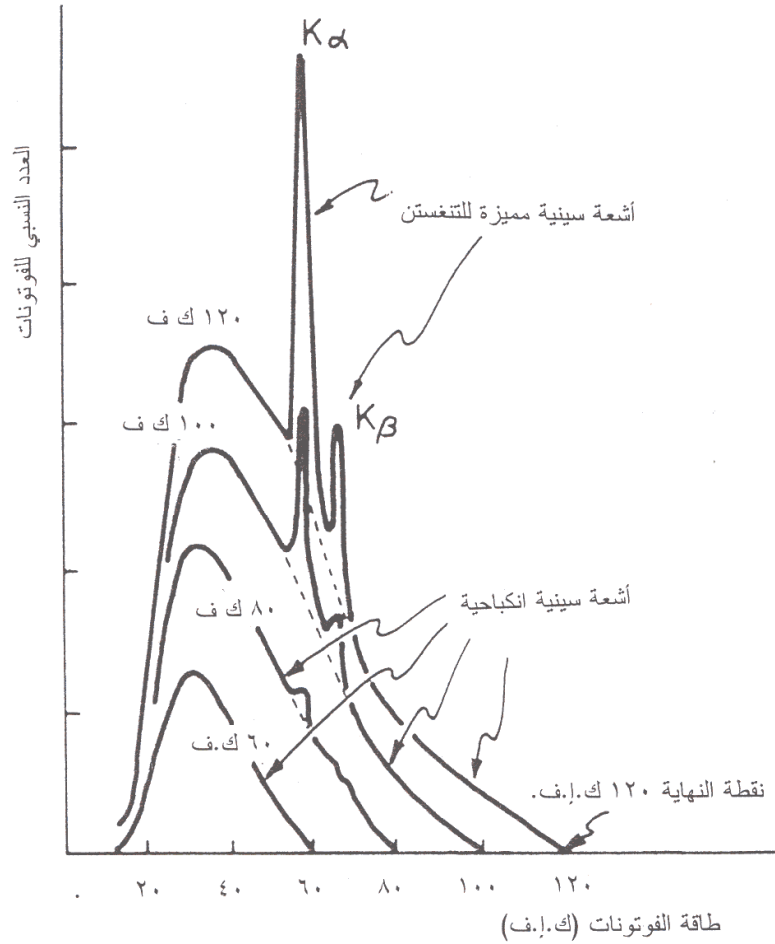
شكل (٩-٢): أطياف الأشعة السينية لجهود تشغيل مختلفة
