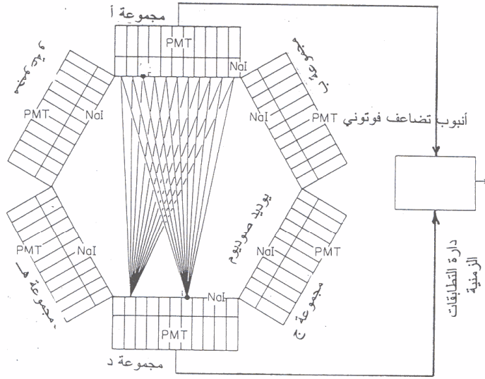
شكل (٩-١١): مخطط المصورة الطموغرافية للانبعاث البوزتروني
