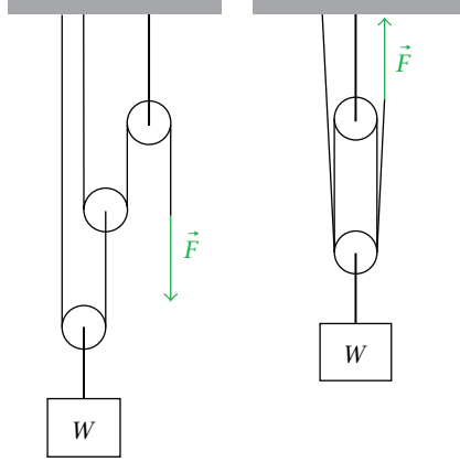
شكل ١٢-٢: كلٌّ من هذين الترتيبين للبكرات يوفر أربعة أضعاف الفائدة الميكانيكية.
