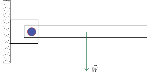
شكل ١٥-٧: قضيب وزنه W مثبت إلى حائط بواسطة مفصل صدى.
