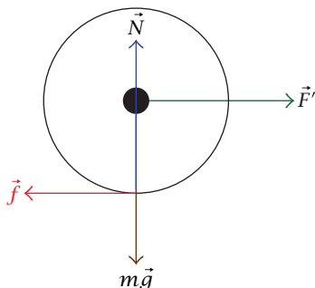
شكل ٨-٢٢: القوى المؤثرة على إحدى عجلات العرب. \vec{F}' هي القوة الأفقية التي يبذلها المحور، و \vec{N} هي مجموع القوى الرأسية التي تبذلها الأرض على المحور.
