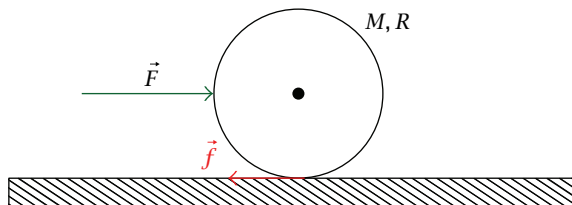
شكل ٨-٢٦: ضُربت كرة بلياردو بقوة دفعية كبيرة بما يكفي لأن تبدأ الكرة الدحرجة بانزلاق في المثال ٨-٨.
