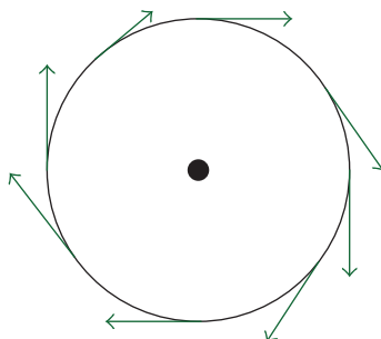
شكل ٨-٢٠: عجلة تدور حول محور خلال مركزها، أو عجلة تتدحرج بطول سطح مسطح كما يُرى من إطار إسناد متحرك مع مركز العجلة، ولها سرعات جزئية كما هو مبين.
