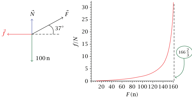
شكل ١٩-٢: مخطط الجسم الحر لمثال ١٢-٢ (أ).
