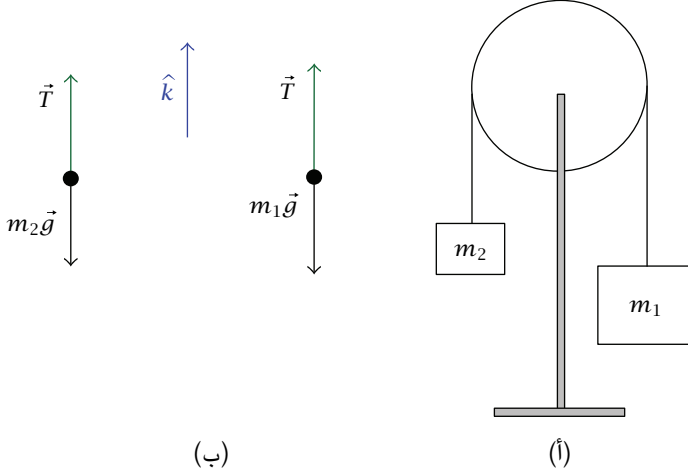
شكل ٣-٥: رسم توضيحي (أ) ومخطط الجسم الحر (ب) للمثال ٣-٤.
