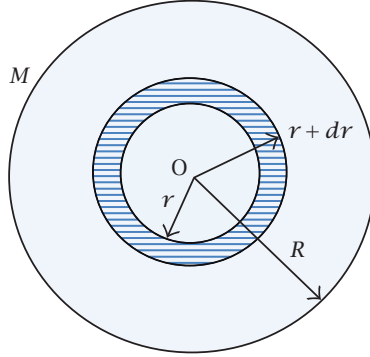
شكل ٨-٧: قرص مسطح نصف قطره R وكتلته M .
