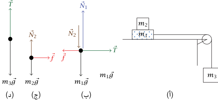
شكل ٩-٣: رسم توضيحي (أ) للمثال ٣-١٠، ومخطط الجسم الحر للكتلة m_1 (ب)، والكتلة m_2 (ج)، والكتلة m_3 (د).
