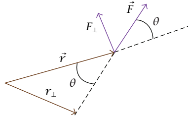
شكل ٣-٧: تعريف F_{\perp} و r_{\perp} .
