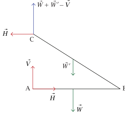
شكل ٧-١٠: مخطط القوة للنظام المركب ABC لمثال ٧-٣.
