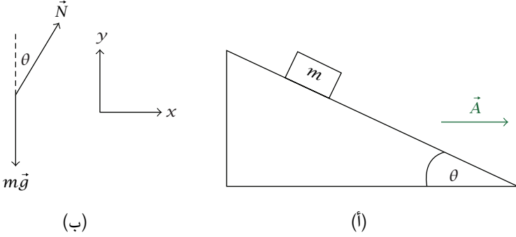
شكل ٣-٢: رسم توضيحي (أ) ومخطط الجسم الحر (ب) للمثال ٣-٢.
