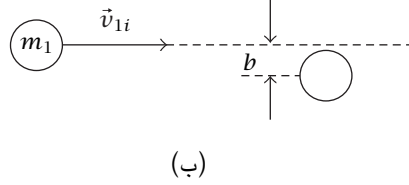
شكل ٥-١٥: تصادم جسمين لهما بارامتر صدم.
