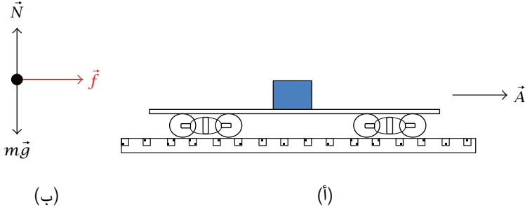
شكل ٨-٣: رسم توضيحي (أ) ومخطط الجسم الحر (ب) للمثال ٣-٩.
