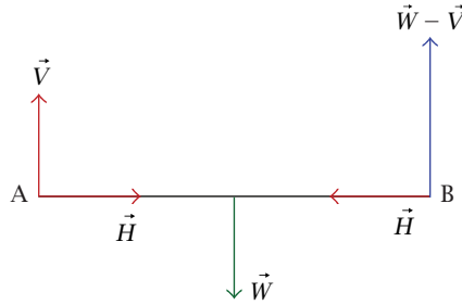
شكل ٧-١١: مخطط القوة للقضيب AB في مثال ٧-٣.
