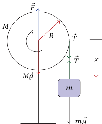
شكل ٨-١١: القوى المؤثرة على القالب والحداثة في مثال ٨-٣.
