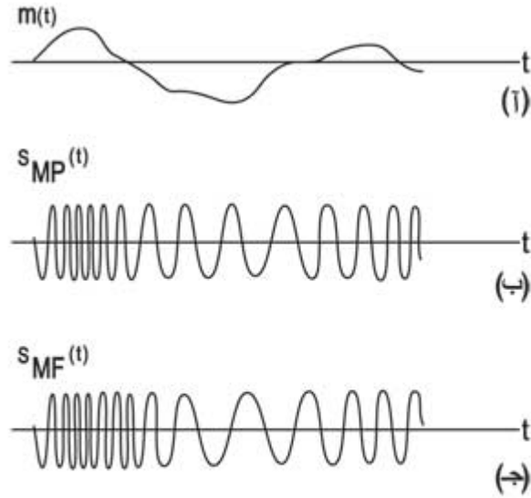
الشكل (٤) شكل الإشارات في حالتها التعديل الطوري والتردد
