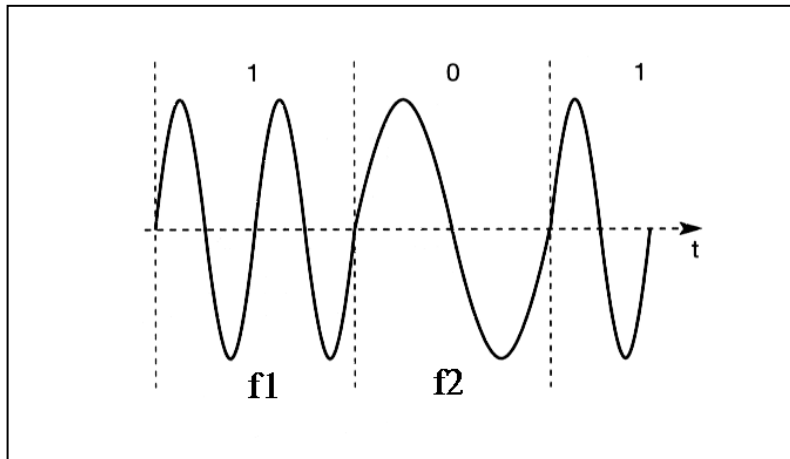
الشكل (٢- ٢) مثال لطريقة تعديل الإزاحة الترددي FSK
