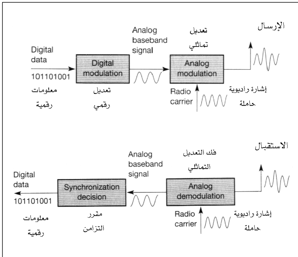
الشكل (٢- ٨) خطوات الإرسال والاستقبال اللاسلكي التماثلي للمعلومات الرقمية.
