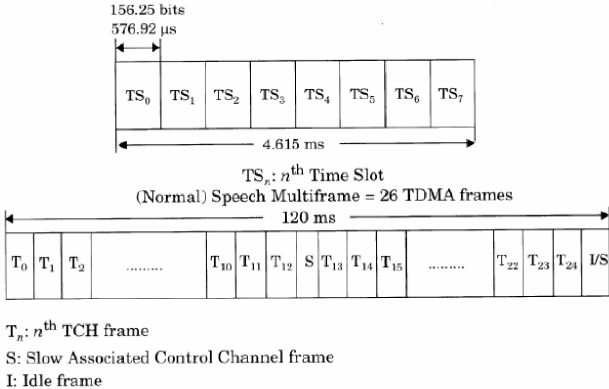
الشكل (٣- ٤) كيفية نقل قنوات الحركة في الرتل
