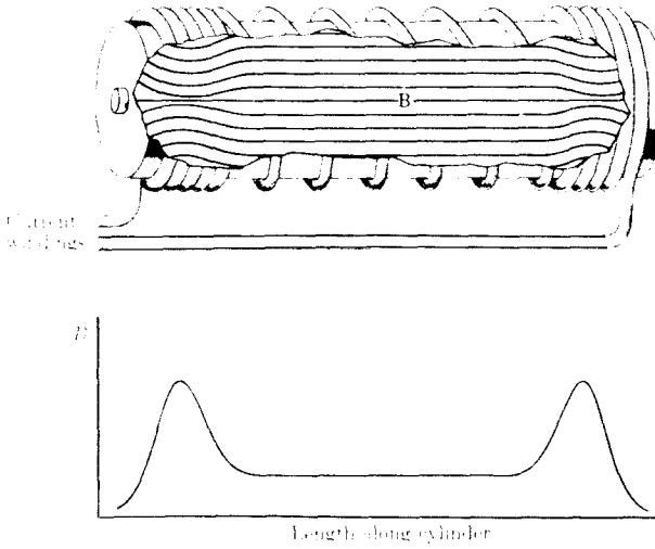
شكل 14-5 منظومة مرآة مغناطيسية .
