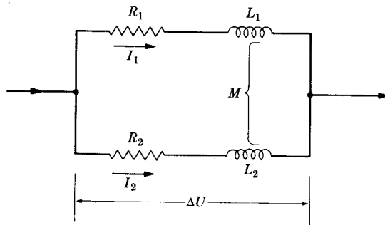
الشكل 4-9 توصيل محثين على التوازي
