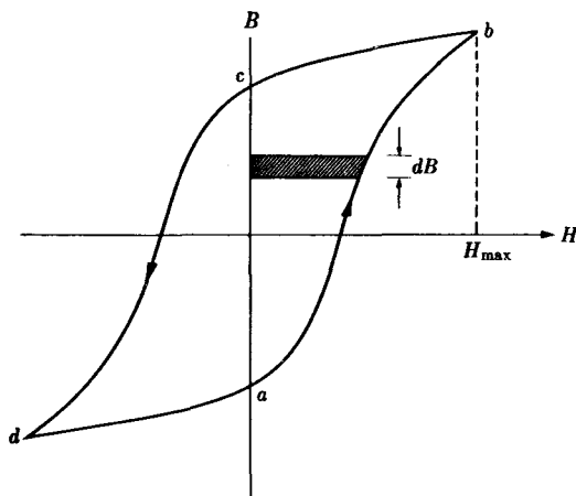
شكل 3-12 الشغل المنجز لوحة الحجم لدورة مادة فيرومغناطيسية .
