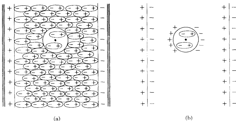
الشكل 5-1 إستبدال العازل خارج التجويف بمنظومة من الشحنتات المقيدة
