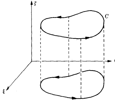
الشكل 8-1 مسقط المنحني C على المستوى \eta - \xi
