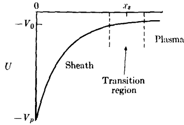
شكل 14-10 . منحنى بياني للجهد كدالة للمسافة عن المحس . bc.
