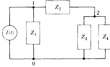
شكل 13-17 . يوضح الشكل طريقة تحميد العقدة لدوائر التيار المتناوب
