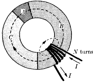
الشكل 10-17 هذه الدائرة المغناطيسية تكافئ الدائرة المغناطيسية المبينة في الشكل 10-16 فيا اذا كانت نفوذية المواد A و B و C عالية .
