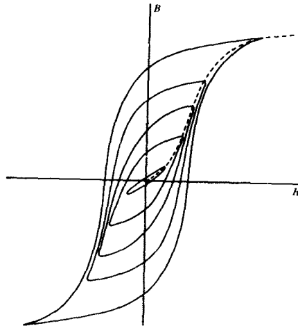
الشكل 10-9 دورة التخلف المغناطيسي الرئيسية وعدد من الدورات الثانوية للتخلف لمادة نموذجية
