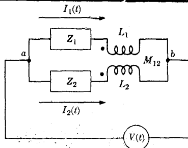
شكل 13-10 . دائرة كهربائية تشتمل على حاثنة متبادلة
