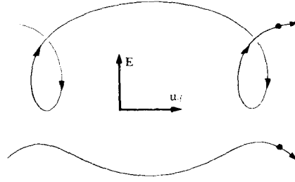
شكل 14-2 . مجالات كهربائية ومغناطيسية متقاطعة . حركة الجسم في مستو عمودي على المجال المغناطيسي . يبين الشكل أيونات متضادة شحناً ذات زخم ابتدائية مختلفة .
