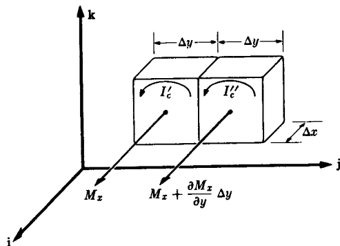
الشكل 10-3 الاستعاضة عن عناصر حجمية لمادة ممغنطة بتيارات دائرية هي I'_c و I''_c .
