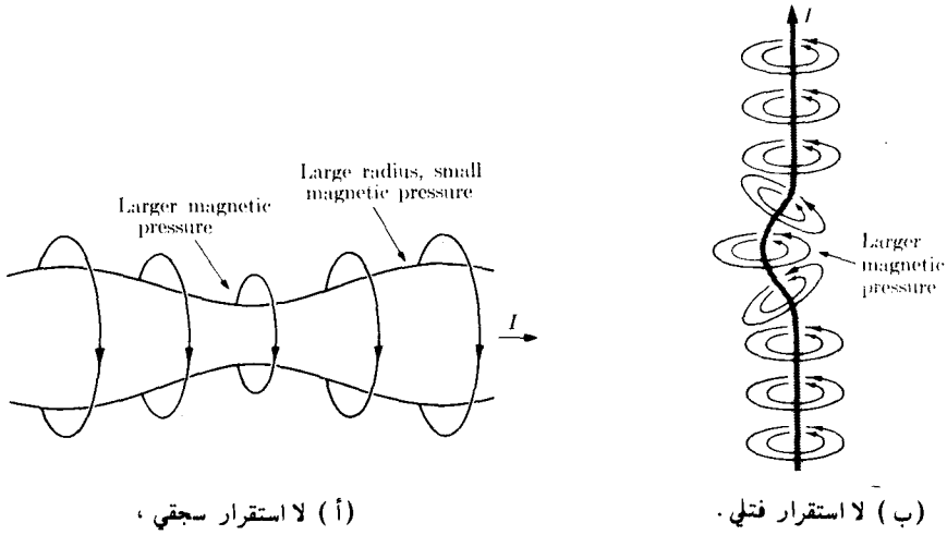
شكل 7-14. الاستقرارية في البلازما المتقلصة :
