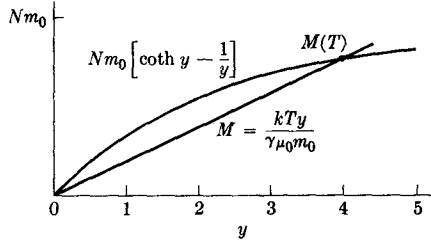
شكل 11-1 . إيجاد التمثيل الذاتي M(T) بمساعدة دالة لانجنج .
