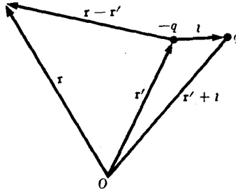
الشكل 2-9 المجال الكهربائي الناشئ عن شحنتين نقطيتين .
