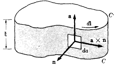
الشكل 6-1 الحجم المتكون من ازاحة مستوي المنحني C في الاتجاه a العمودي على المساحة
