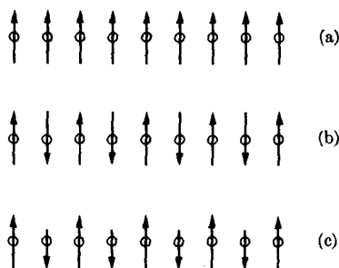
شكل 6-11 . تمثيل تخطيطي لبروم ذرية في تراكيب برمية مرتبة ، (a) فيرومغناطيسي ، (b) لا فيرومغناطيسي ، (c) فيريمغناطيسي .
