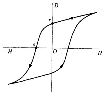
الشكل 7-10 دورة نموذجية للتخلف المغناطيسي في مادة فيرومغناطيسية .
