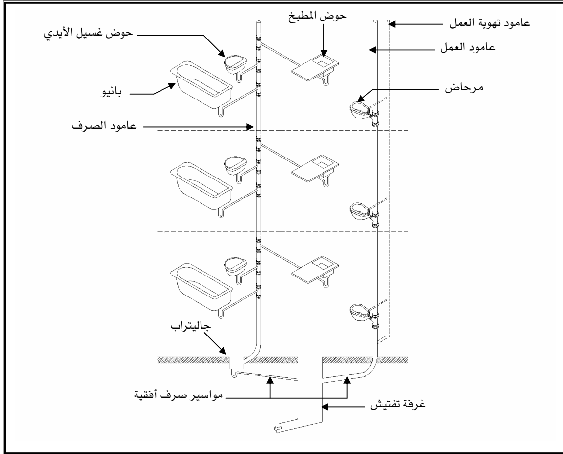
شكل (١- ١٧) : النظام المعدل لماسورتين مع تهوية أفرع ماسورة العمل
