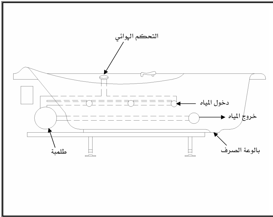
شكل ( ١ - ٥٠ ) : أحد أنواع البانيوهات ويسمى "جاكوزي" ، و يلاحظ حركة المياه داخله
