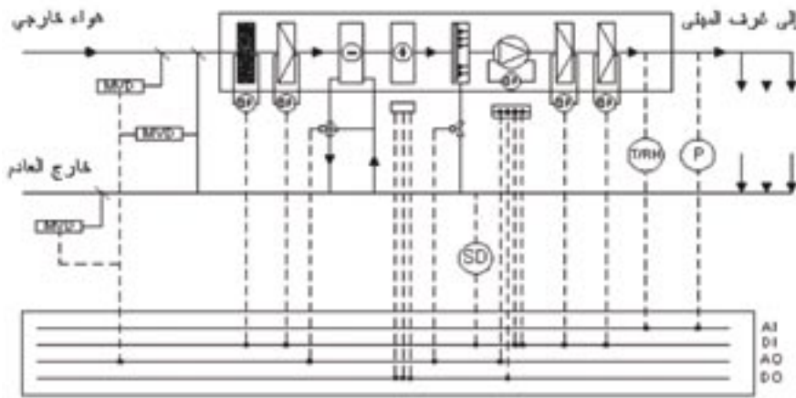
شكل ٩-٨ مخطط نمطي لنظام تحكم رقمي لوحدة معالجة هواء
