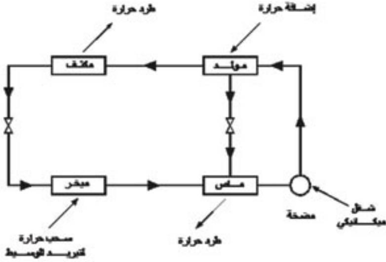
شكل ١-٣ توضيح الفكرة الأساسية للتبريد بامتصاص البخار
