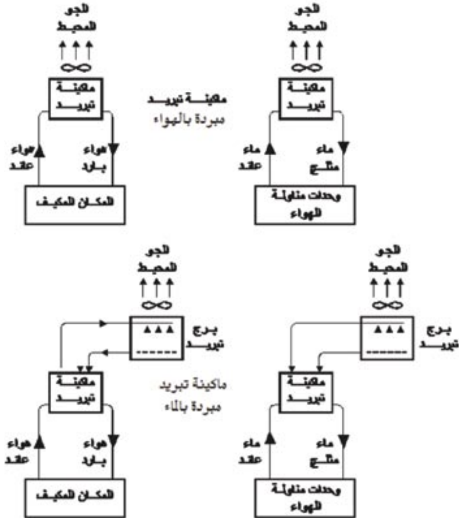
شكل ٦-١٠ البدائل المختلفة لطرق عمل ماكينات التبريد: ماكينات مبردة بالهواء (أعلى الرسم)، وماكينات مبردة بالماء (أسفل الرسم)
