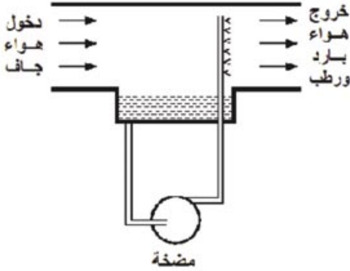
شكل ١-٤ الفكرة الأساسية لتبريد الهواء بالتبخير
