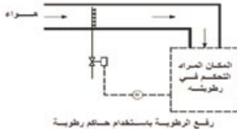
شكل ٩-٣ التحكم في الرطوبة
