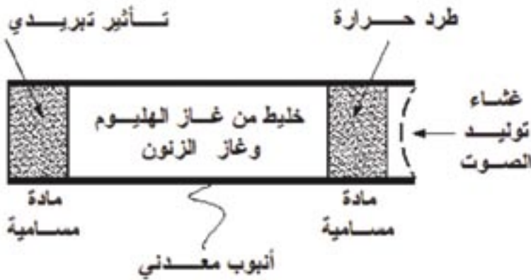
شكل ٦-٤ الفكرة الأساسية للتبريد الصوت حراري
