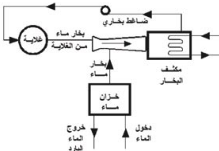
شكل ٣-٤ التبريد باستخدام نفثات بخار الماء
