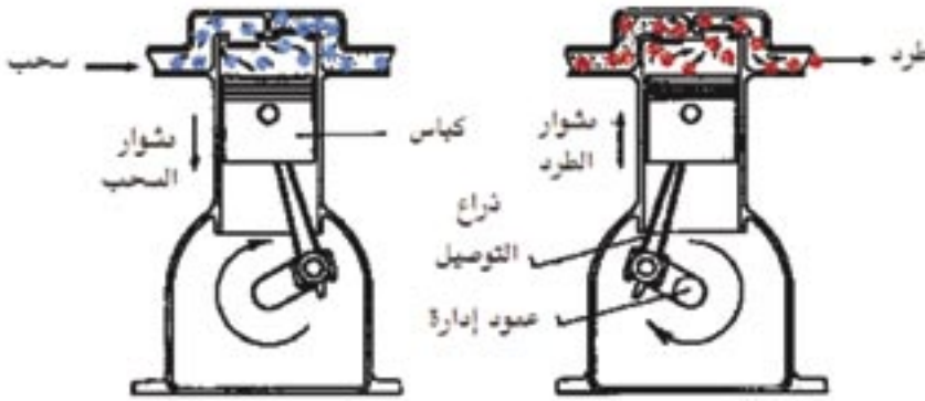
شكل ٩-٢ رسم توضيحي للمضامط الترددي
