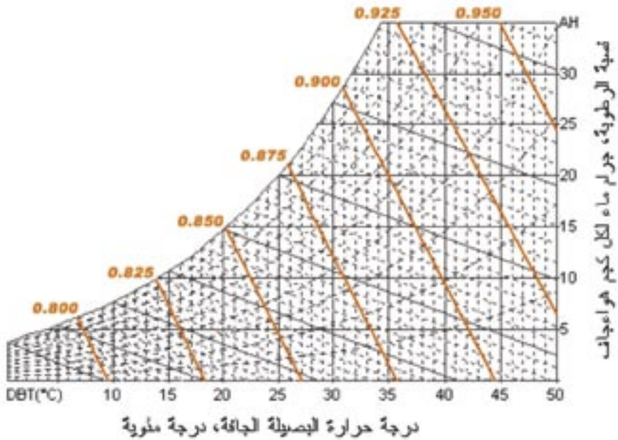
شكل ٢-٥ الخريطة السيكمومترية لخواص الهواء الرطب
