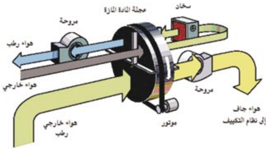
شكل ٨-٢ عجلة المادة المازة لتجفيف الهواء
