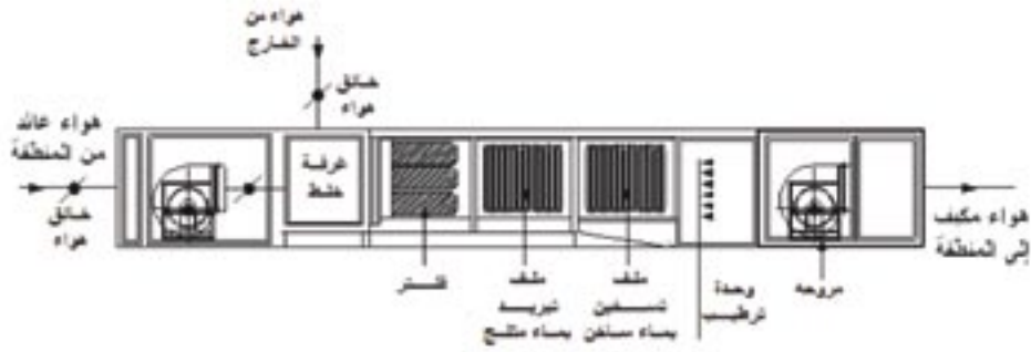
شكل ٣-٦ نموذج لوحدة مناولة هواء بها مروحتان وملف تبريد وملف تسخين ومرطب
