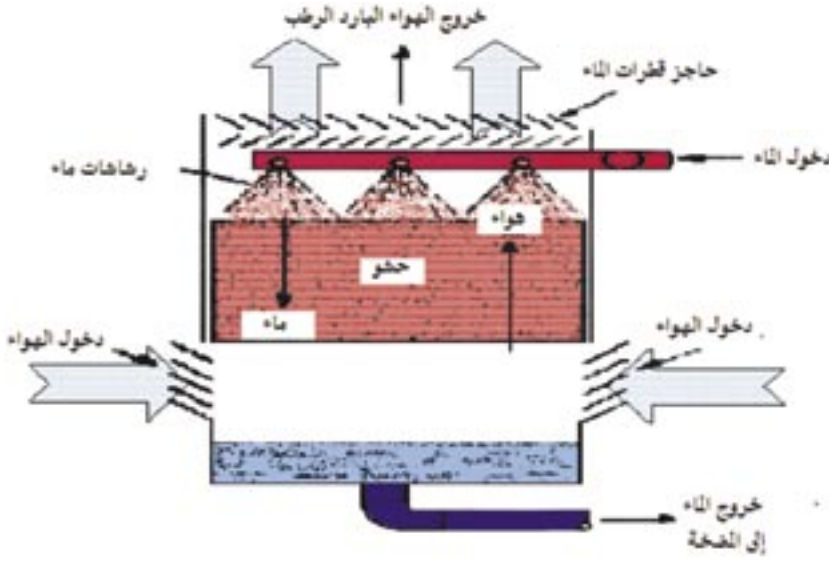
شكل ٨-١ مآكينات تبريد الهواء بالتبخير
