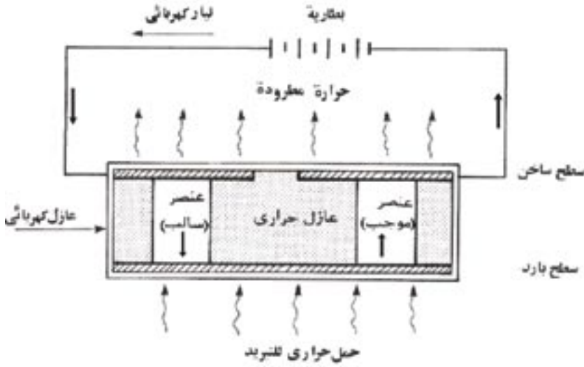
شكل ٢-٤ طريقة عمل التبريد الكهروحراري
