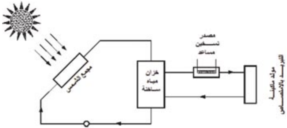
شكل ٣-٥ استخدام الطاقة الشمسية لتشغيل ماكينة تبريد بالامتصاص
