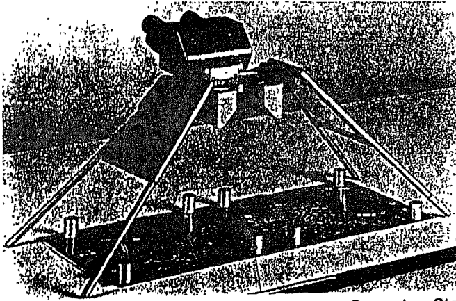
شكل (٣٧): جهاز استريوسكوب ذو المرايا
