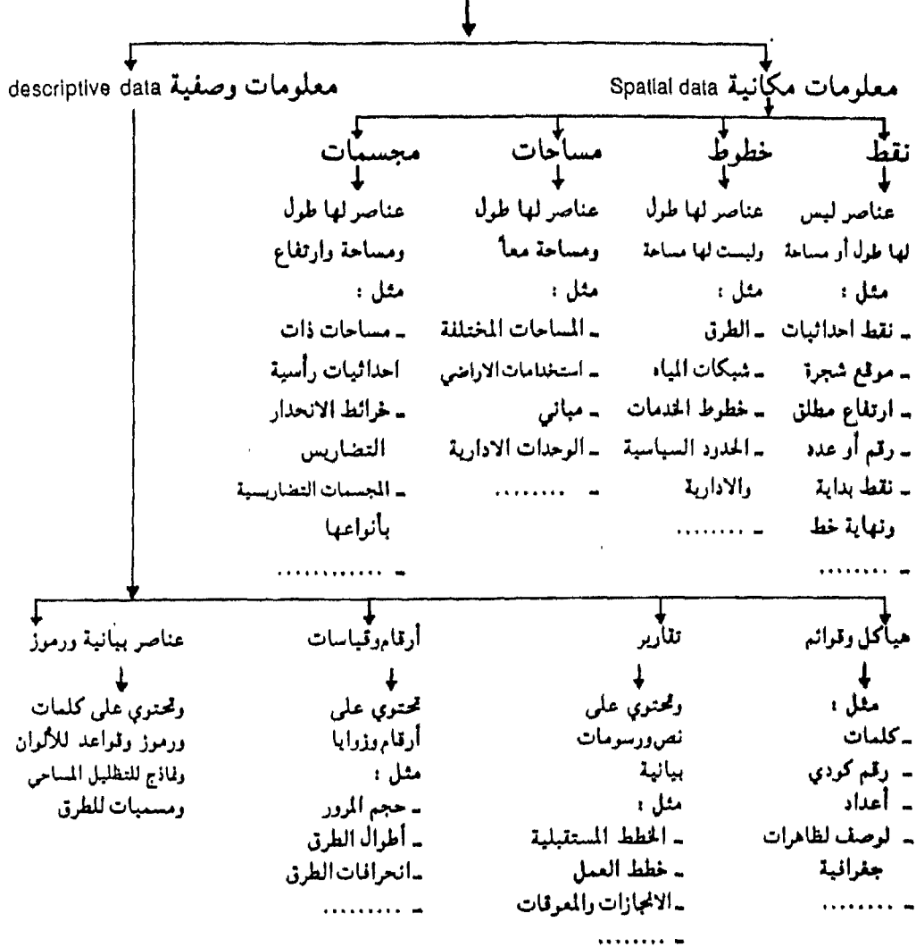
شكل (١٤) : يوضح المكونات الأساسية لقاعدة المعلومات الجغرافية
