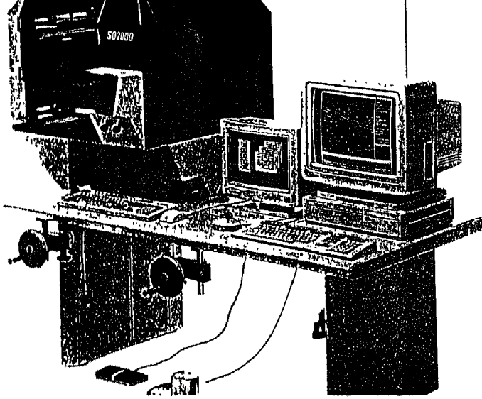
شكل (٤٣): جهاز استريوبلوتر
