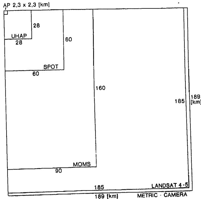
شكل (٤٥): رسم تخطيطي للمقارنة بين أحجام المرئيات المختلفة
