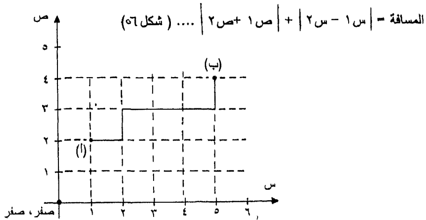
شكل (٥٦): طريقة مانتاتن المترية لحساب المسافة بين النقط
