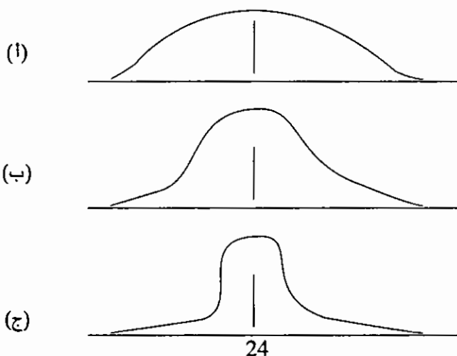
شكل (5) ثلاثة توزيعات للدرجات لها نفس المتوسط لكن تشتت درجاتها مختلف
