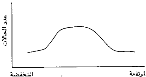
شكل (8) منحنى مفلطح
