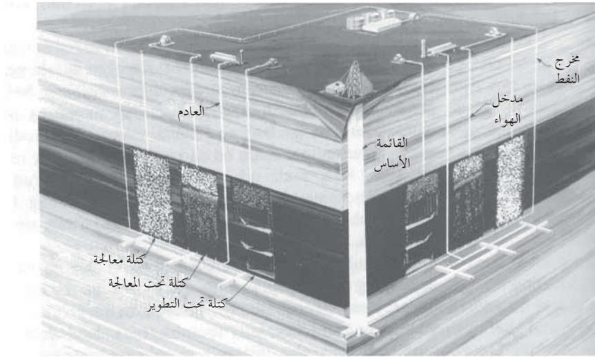
الشكل ج-13: استرداد نفط السجّيل موقعياً
