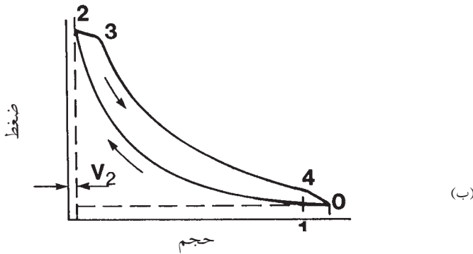
الشكل 19.3 دورة الديزل لمحرك احتراق داخلي
