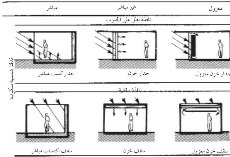
الشكل 2-11: التدفئة الشمسية السكونية (السلبية)
