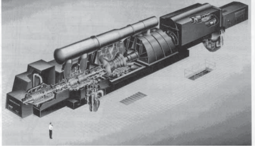
الشكل 13.3 مولد توربيني بخاري كبير
