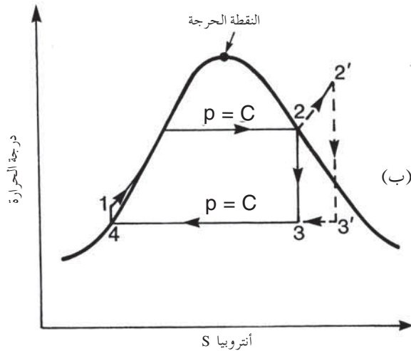
الشكل 9-A: شكل دورة رانكين البيانية.
