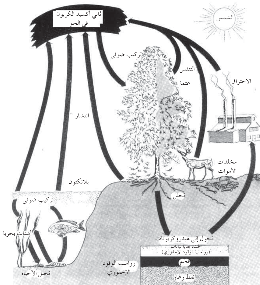
الشكل 9-6: دورة الكربون
