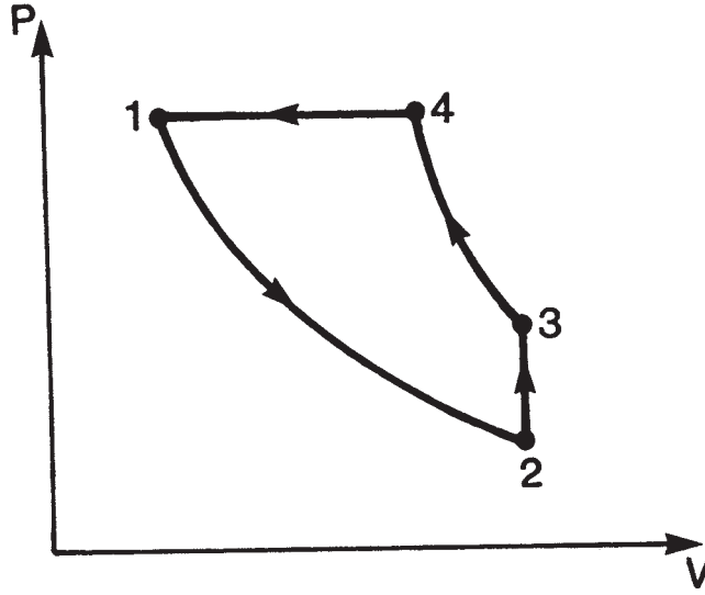
الشكل A-5: دورة ثيرموديناميكية
