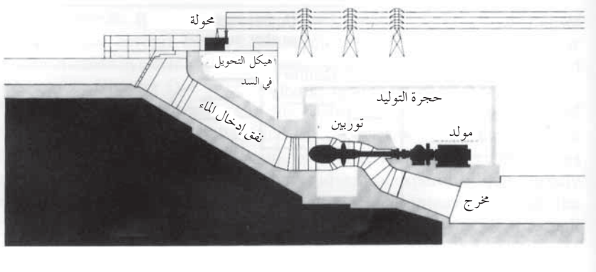
الشكل 12.3 مخطط محطة توليد كهرومائي. تقدمة: City of Seattle. Light Dept.
