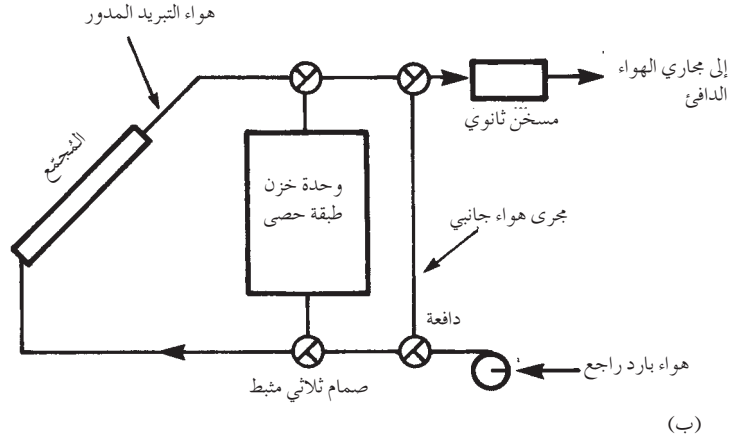
الشكل 3-11: أنظمة شمسية - حرارية فاعلة. (أ) نظام ماء ساخن منزلي. (ب) نظام منزلي للتدفئة بالهواء الساخن المصدر: U.S. Dept. of Energy (1981)
