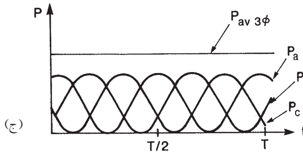
الشكل 14-A: أشكال موجات مولد التيار المتناوب عبر الزمن (أ) فيض القطب المغنطيسي «مقابل الزمن». (ب) الفولتيات ثلاثية الأطوار مقابل الزمن. (ج) القدرة ثلاثية الأطوار مقابل الزمن.
