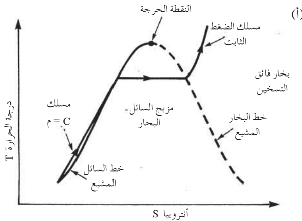
الشكل 8-A: الشكل T S- للماء والبخار.
