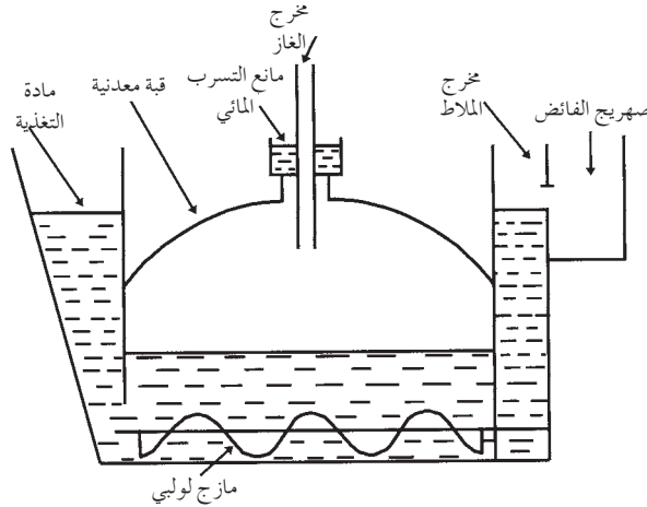
الشكل 11-14: جهاز هضم الغاز الحيوي المستخدم في العالم الثالث. مقتبس من Dun, 1986.
