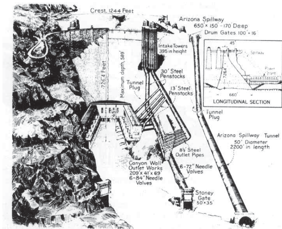
الشكل 11.3 سد هوفر - مصنع كهرومائي ملحق
