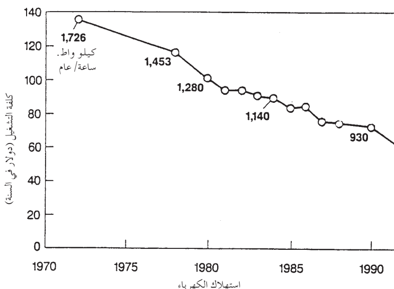
الشكل 5.4 كلفة التشغيل السنوية واستهلاك الكهرباء لثلاجات جديدة في الولايات المتحدة مقتبسة من Gellings and Lovins Fickett، (انظر المراجع، الفصل التاسع).
