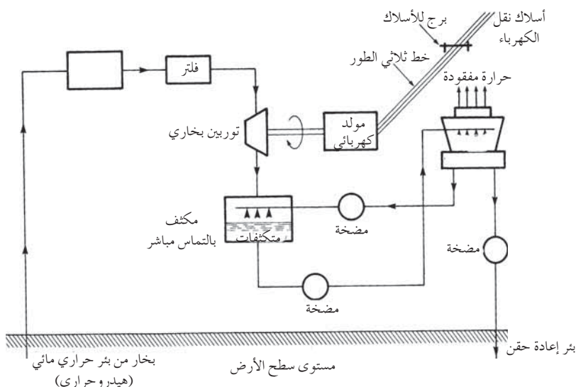
الشكل ج-17: محطة قدرة كهربائية هيدروحرارية - من نوع البخار الجاف المباشر
