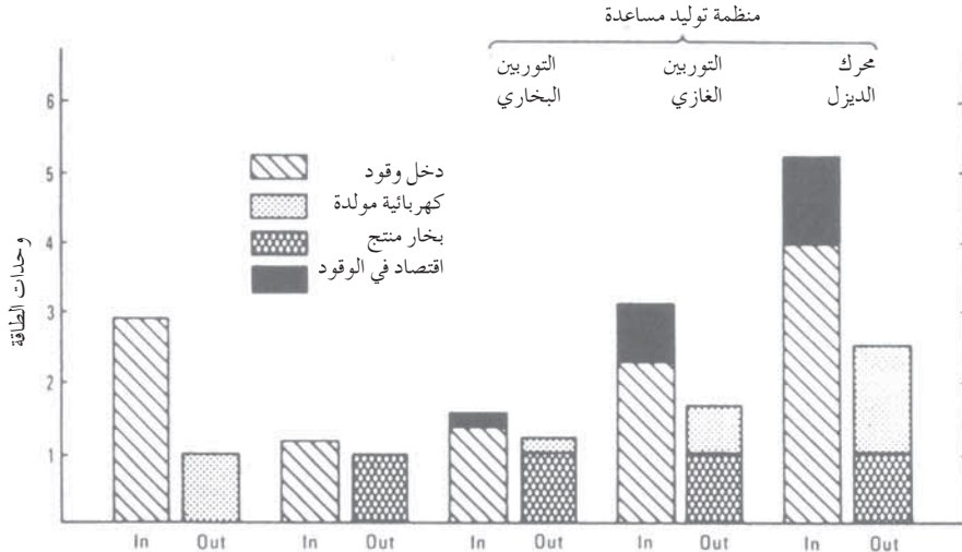
الشكل ج-4: مقارنة الأداء - لأنظمة التوليد المزدوج. مدخلات ومخرجات الطاقة لعينات من تكنولوجيا التوليد المزدوج.
