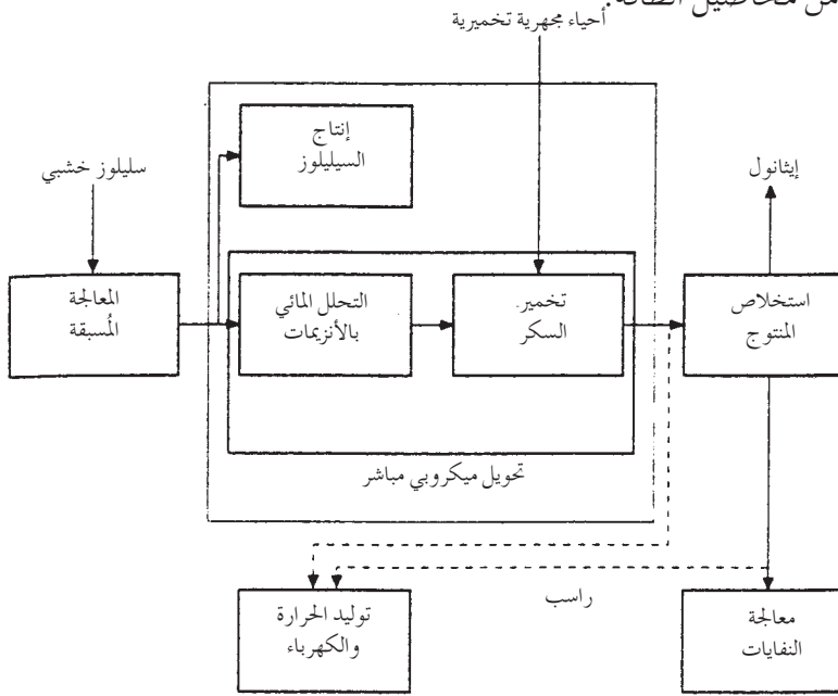
الشكل 11-13: التسكير والتخمير المتزامنين ملاحظة: السيليلاز هو إنزيم يساعد في التحلل المائي للسيليلوز. مقتبس من: Johannson [et al.], 1993.
