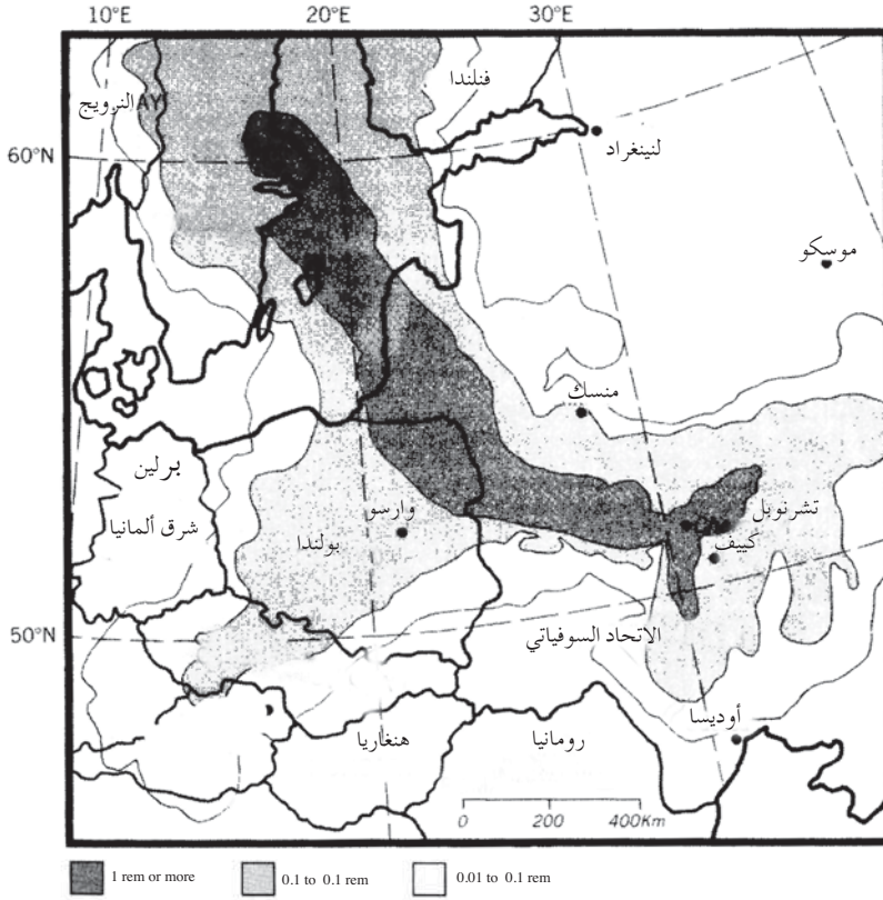
الشكل 7-14: تقديرات جرعة الدرقية التي جرى استنشاقها بعد أربعة أيام من حادث تشرنوبل. طبعت بإذن من Bulletin of the Atomic Scientists وهي مجلة للعلوم والعلاقات الدولية، حقوق الطبع 1986 من قبل. Foundation for Nuclear Science, 6042 South Kimbark Avenue, Chicago, Illinois 60637.
