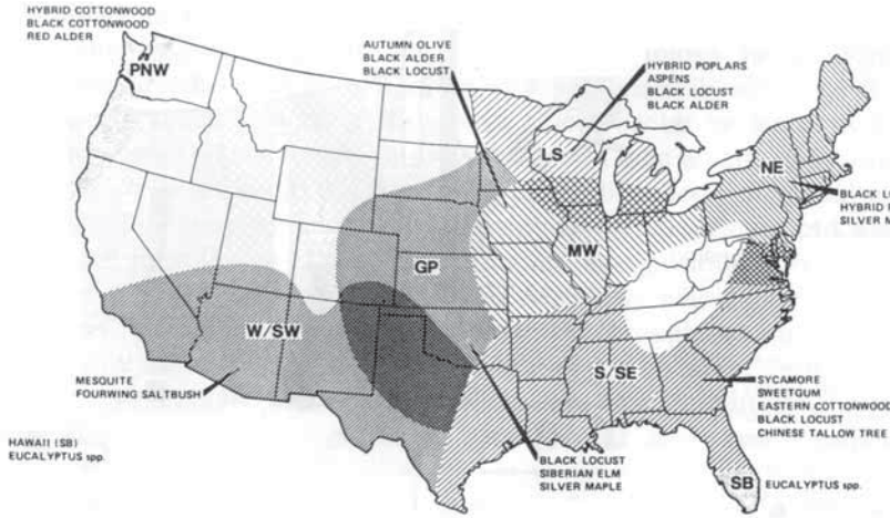
الشكل 11.2: مواقع إمداد الخشب كثافة في الولايات المتحدة الأمريكية المصدر: بور وآخرون (Boer, et al. , 1986)
