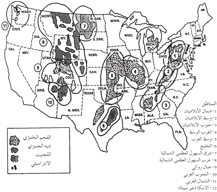
الشكل 3-6: التوزيع المناطقي لاحتياطيات الفحم في الولايات المتحدة
