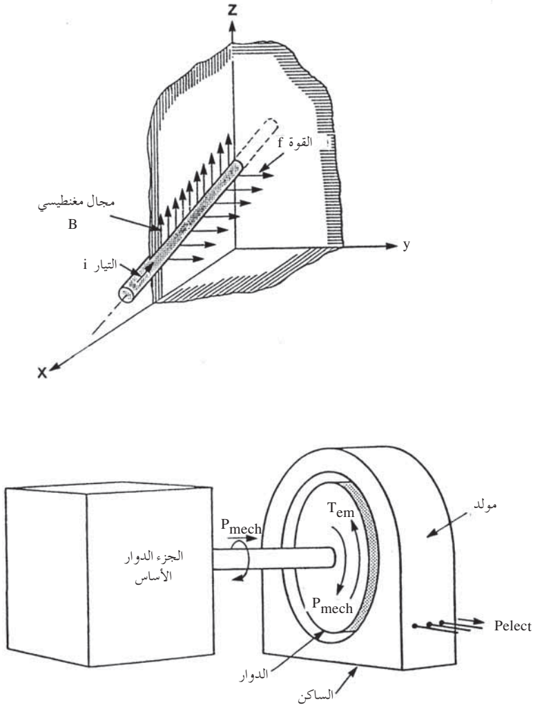
الشكل A-15: التفاعل البيني للمحرك الأولي/ المولد (أ) القوة المغناطيسية في موصل حامل للتيار (ب) عزم اللي والدوران. مقتبس من: (Elgerd (1978)
