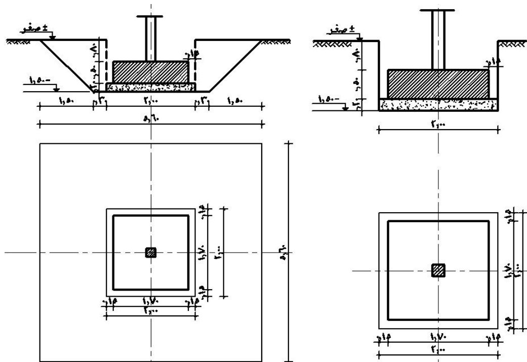
شكل رقم (٧ - أ) الحصر بطريقة قياس المهندس شكل رقم (٧ - ب) الحصر بطريقة قياس الماثل
