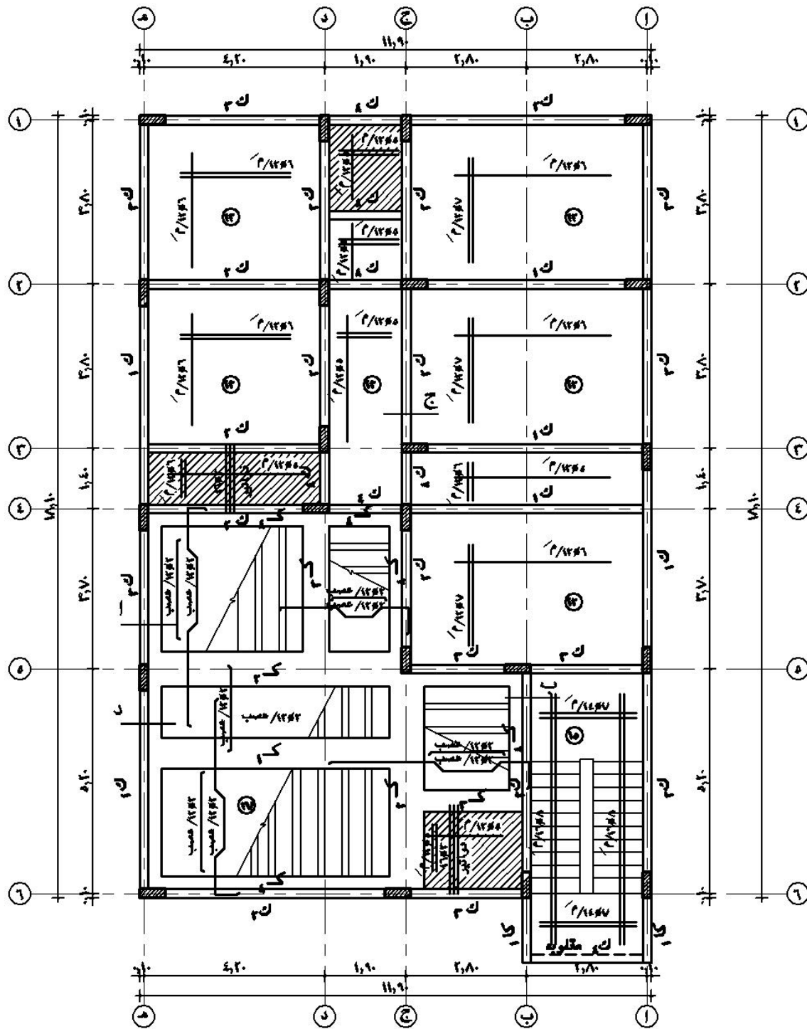
تسليح سقف الدور الأرضي والاول
