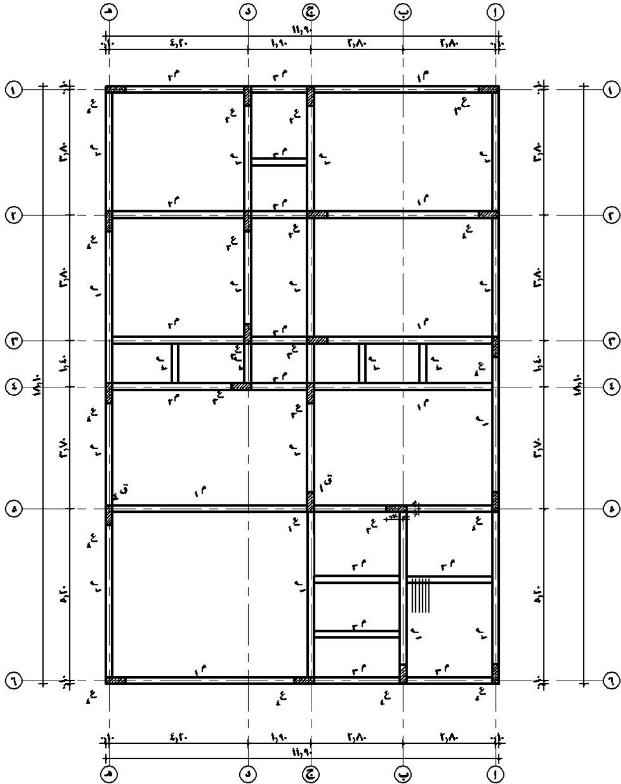
مسقط افقى للميدات
