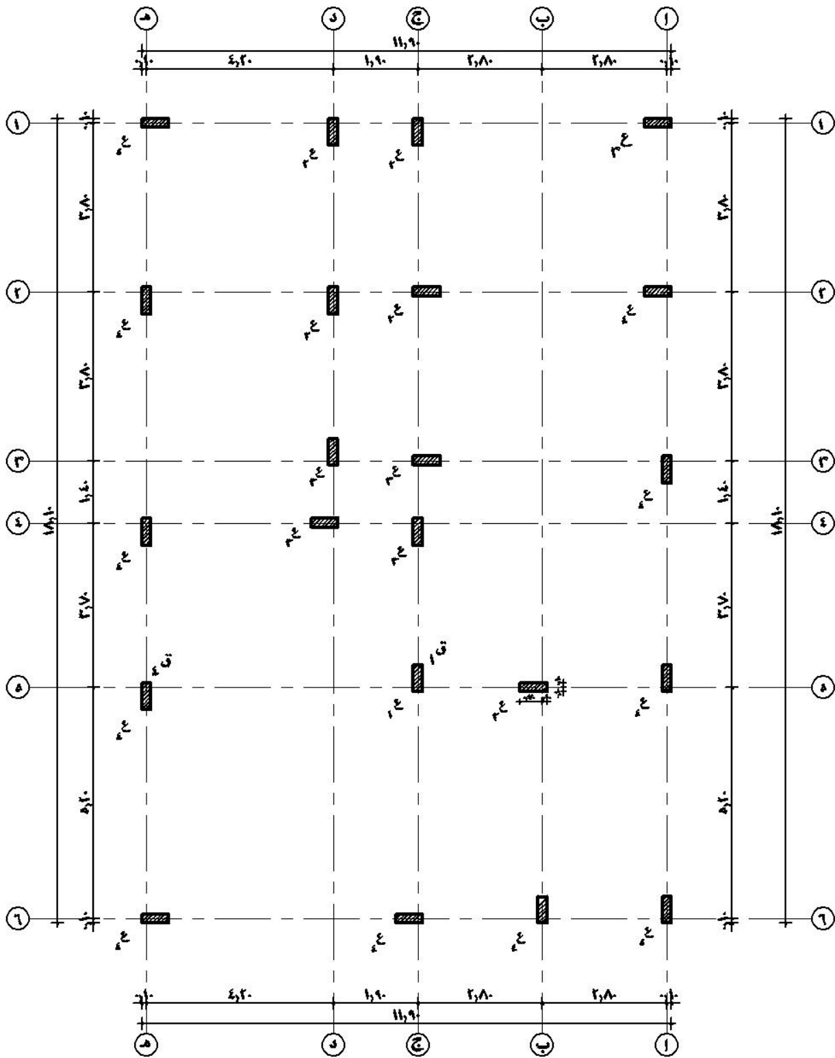
لوحة الأعمدة
