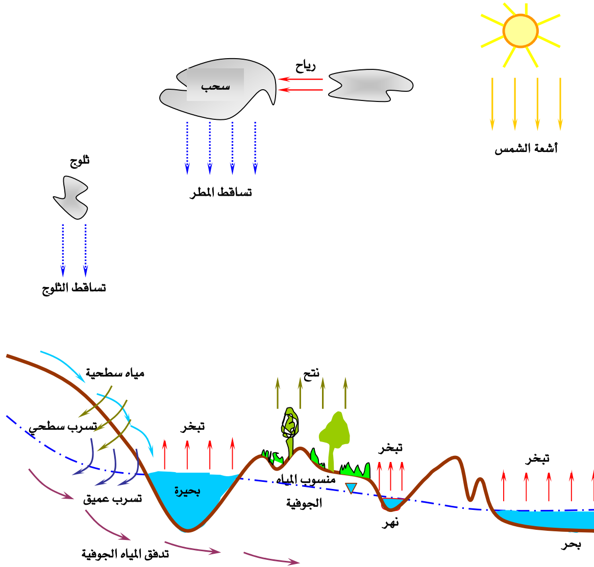
الشكل (٦-١): الدورة الهيدرولوجية للماء
