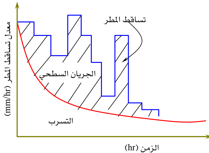
الشكل (٩- ١): نموذج لمنحنى مائى
