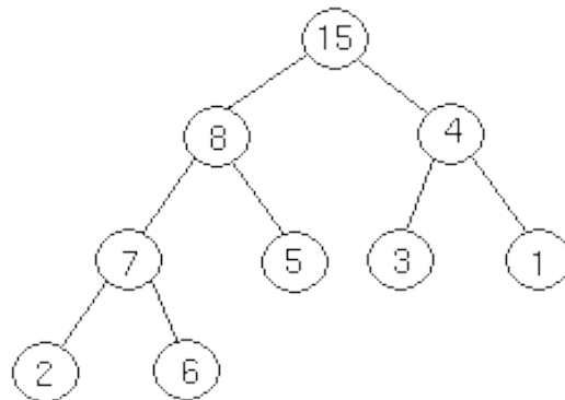
شكل (3-14) مثال للإجراء Heapify (4)
