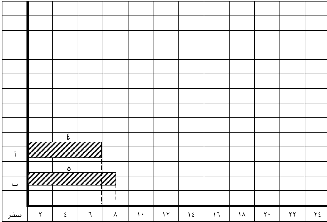
شكل (٣- ١٢) : تجميع أكثر من نشاط في حدود أعداد العمالة المسموح بها
